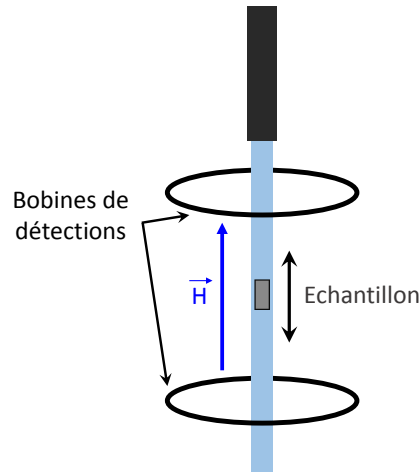
FIGURE 2.10 – Représentation schématique du principe de fonctionnement du VSM.
