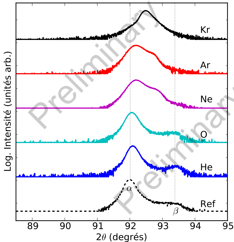
FIGURE 3.18 – Diffractogrammes des couches minces de MnAs irradiées avec une fluence similaire, 10^{13} ions \text{cm}^{-2} , mais avec des ions de masse différente (résultats préliminaires).
