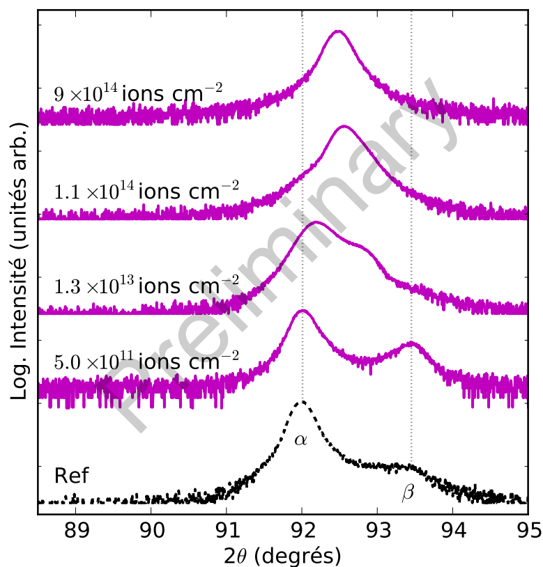
FIGURE 3.26 – Diffractogrammes des couches minces de MnAs irradiées avec différentes fluences d'ions néon (résultats préliminaires).
