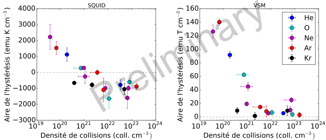
FIGURE 5.1 – Évolution de l'aire de l'hystérésis extraite des mesures SQUID ( M = f(T) ) et VSM ( M = f(H) ) en fonction de la densité de collisions dans la couche mince (résultats préliminaires).
