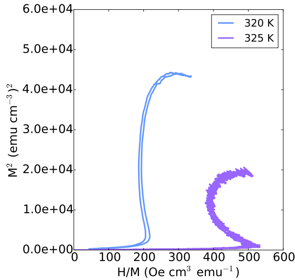
FIGURE 5.3 – Courbes d’Arrott d’un échantillon appartenant au régime d’irradiation 1 (résultats préliminaires).
