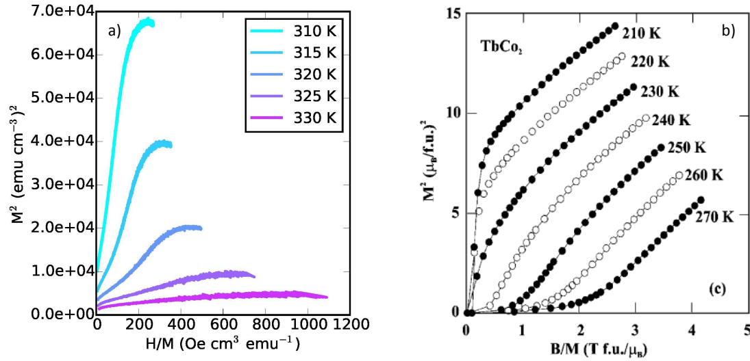
FIGURE 5.6 – Courbes d’Arrott d’un échantillon irradié dans des conditions correspondant au régime 2 a) (résultats préliminaires). Courbes d’Arrott typique d’un matériau présentant une transition de phase de deuxième ordre b).
