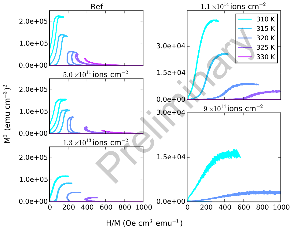
FIGURE 3.25 – Courbes d'Arrott pour différentes fluences, obtenues à des températures proches de la température de transition de phase (résultats préliminaires).
