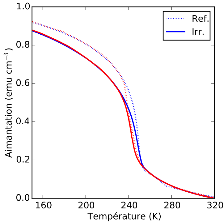
FIGURE 5.13 – Évolution de l'aimantation en fonction de la température à 1 T de la poudre de référence et la poudre irradiée avec une fluence de 3.5 \times 10^{14} ions \text{cm}^2 ( \pm 50\% ) (résultats préliminaires).
