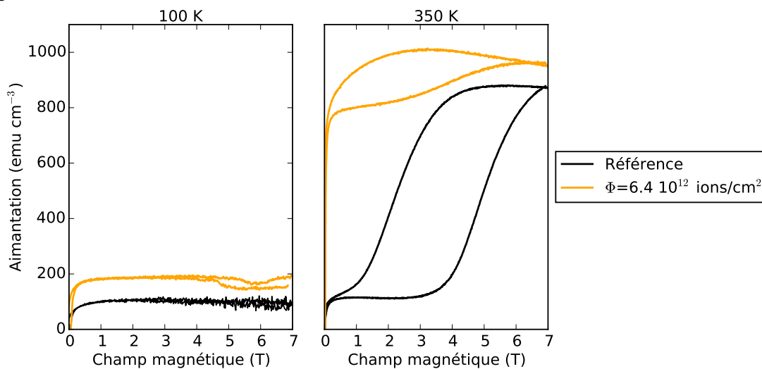
FIGURE 4.18 – Aimantation en fonction du champ magnétique appliqué acquise à 100 K et 350 K sur l'échantillon de référence et irradié.
