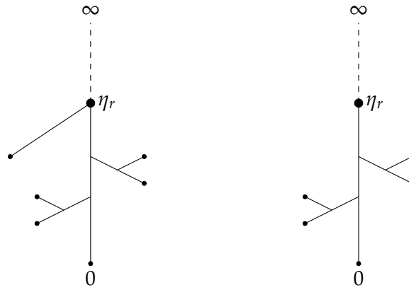
FIGURE 2.1 – Disques fermés
