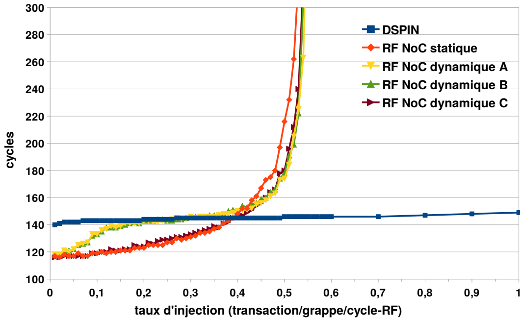
Figure 6.12 – Latence moyenne des communications 1 vers 1 pour un CMP 32 \times 32
