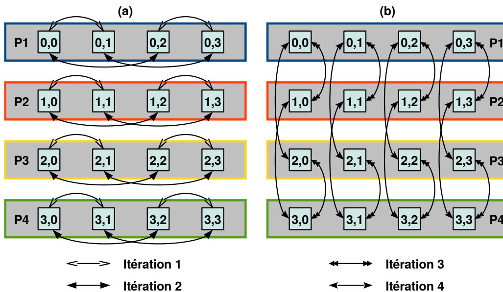
Figure 6.10 – Combinaisons réalisées lors du calcul de la FFT d'une matrice 4 \times 4 stockée par lignes dans la mémoire locale de 4 processeurs
