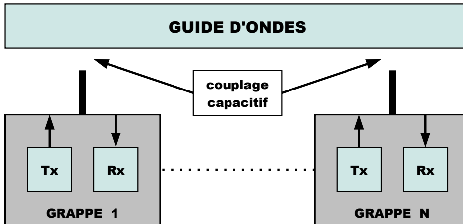
Figure 4.8 – Guide d’ondes
