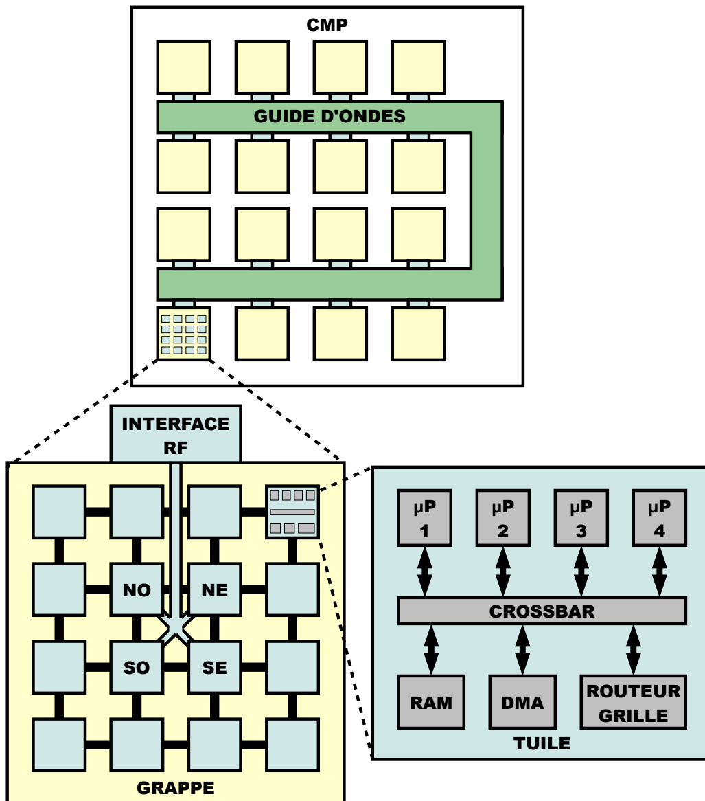
Figure 4.1 – Organisation hiérarchique du CMP et topologie du NoC pour une configuration de 16 grappes de 16 tuiles de 4 cœurs
