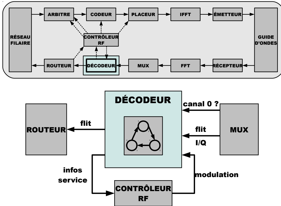
Figure 4.12 – Décodeur
