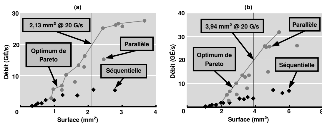
Figure 6.7 – Surface (mm 2 ) en fonction du taux d'échantillonnage (Giga Échantillons par seconde) de FFT 1024 (a) et 4096 (b) points pour une implémentation ASIC 65 nm ( extrait de [Milder et al., 2012] )
