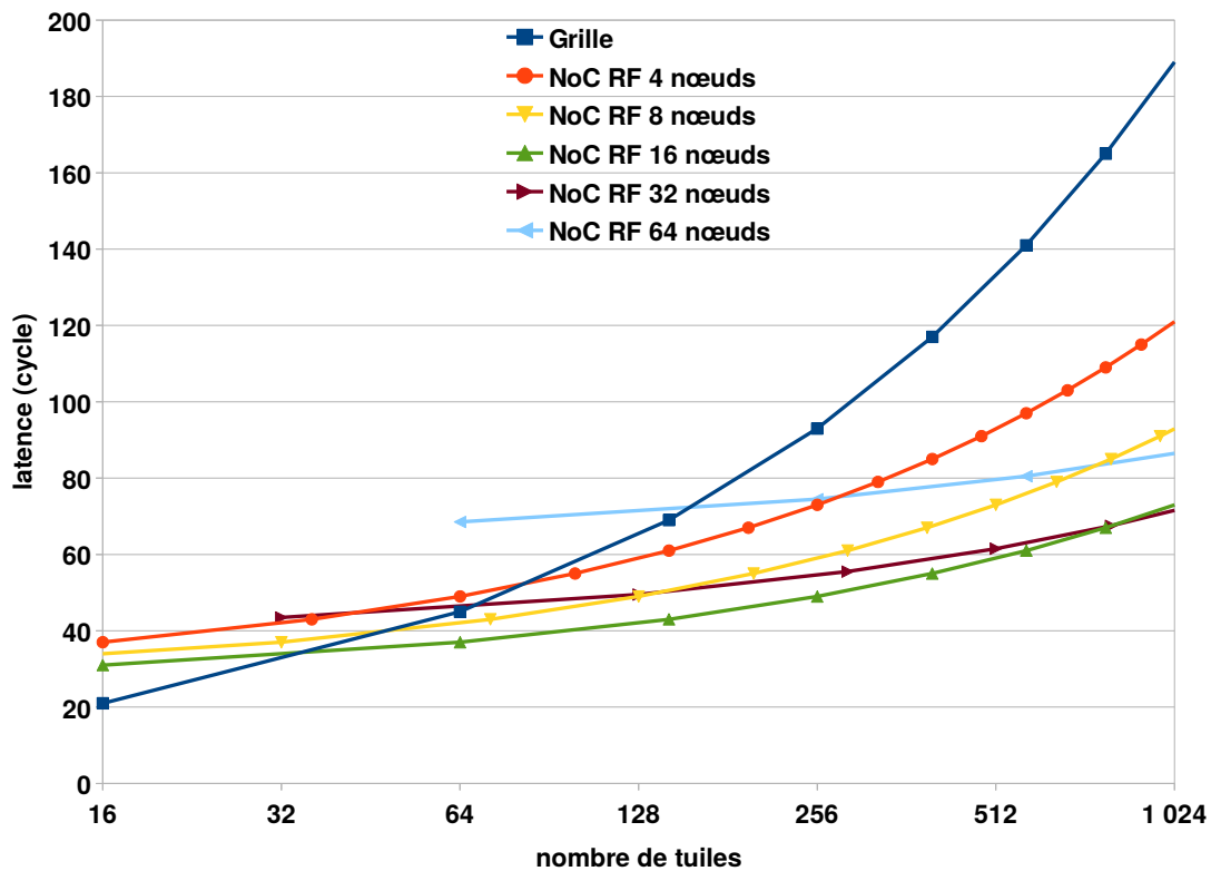
Figure 6.4 – Latence maximale du broadcast d'un FLIT sur une grille et sur un NoC RF à un nombre fixe de 16 canaux de communication
