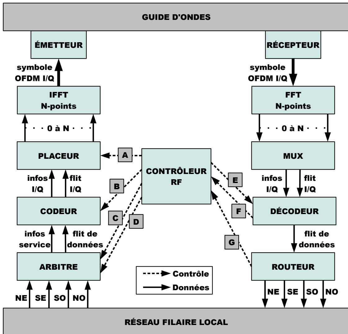
Figure 4.2 – Schéma fonctionnel de l'Interface RF
