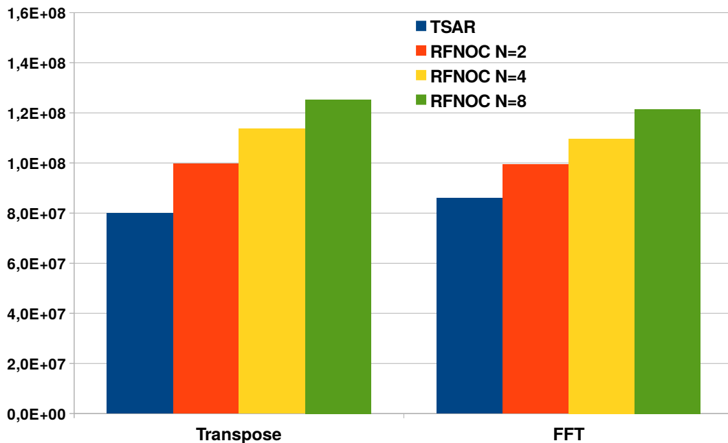
Figure 6.11 – Temps d'exécution total sur un CMP de 8 \times 8 tuiles
