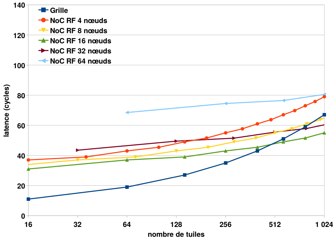
Figure 6.2 – Latence moyenne du transfert point à point d'un FLIT sur une grille et sur un NoC RF ayant un nombre fixe de 16 canaux de communication
