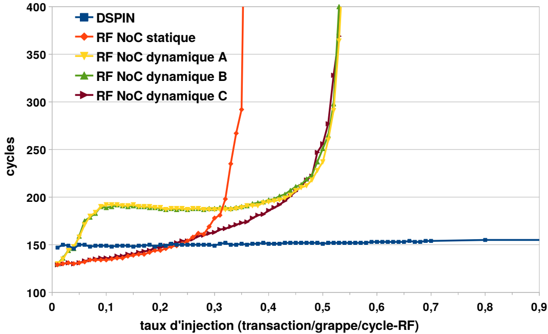
Figure 6.16 – Latence moyenne des communications pour un profil mixte dans un CMP 32 \times 32
