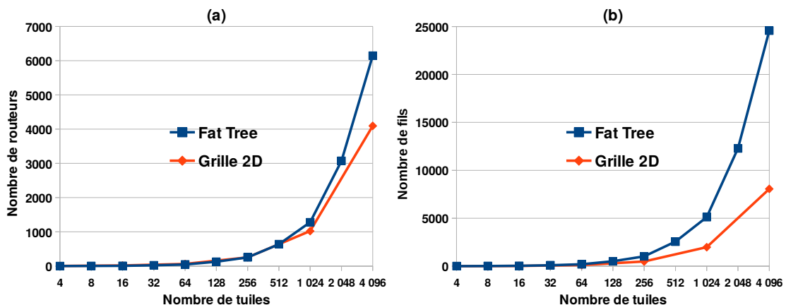
Figure 3.1 – Nombre de routeurs (a) et de connexions filaires (b) dans un CMP utilisant un Fat Tree ou une grille 2D
