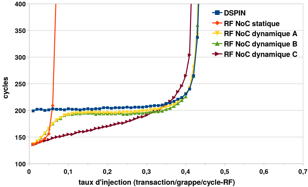
Figure 6.13 – Latence moyenne des communications N vers 1 pour un CMP 32 \times 32
