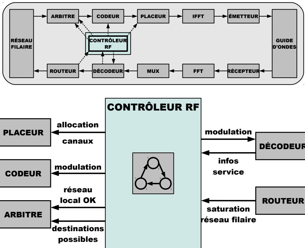
Figure 4.14 – Contrôleur RF
