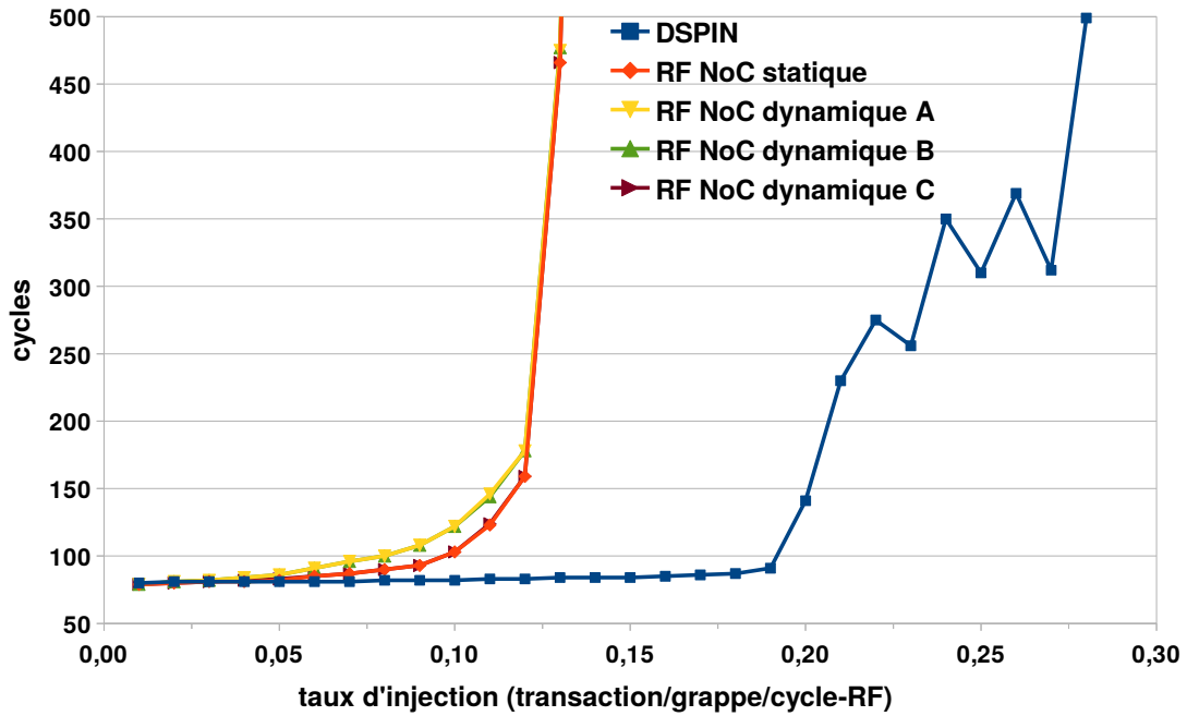
Figure 6.15 – Latence des communications de type broadcast sans réponse pour un CMP 32 \times 32
