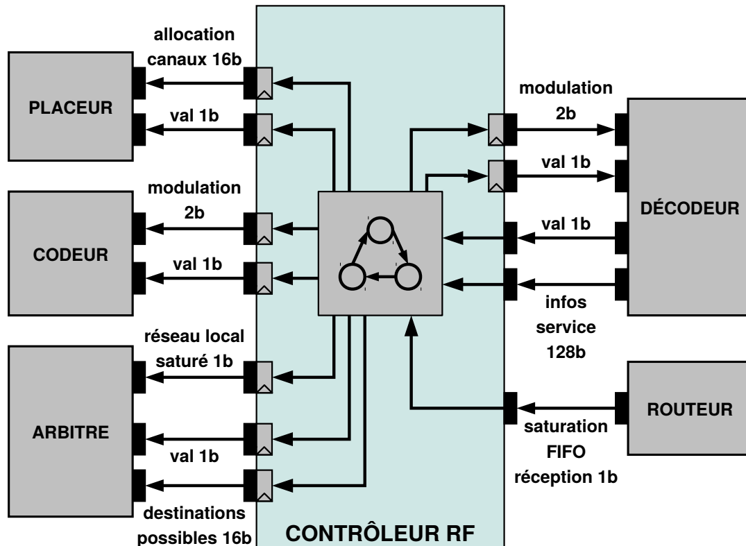
Figure 5.10 – Modèle du contrôleur RF
