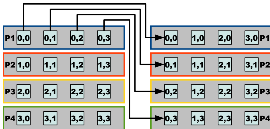
Figure 6.9 – Transposition d'une matrice 4 \times 4 stockée dans la mémoire locale de 4 processeurs
