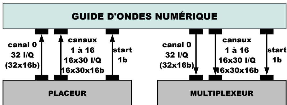
Figure 5.6 – Modèle du guide d'ondes numérique
