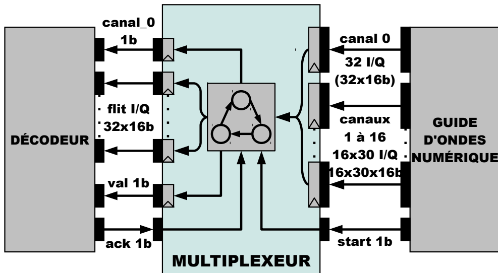
Figure 5.7 – Modèle du multiplexeur
