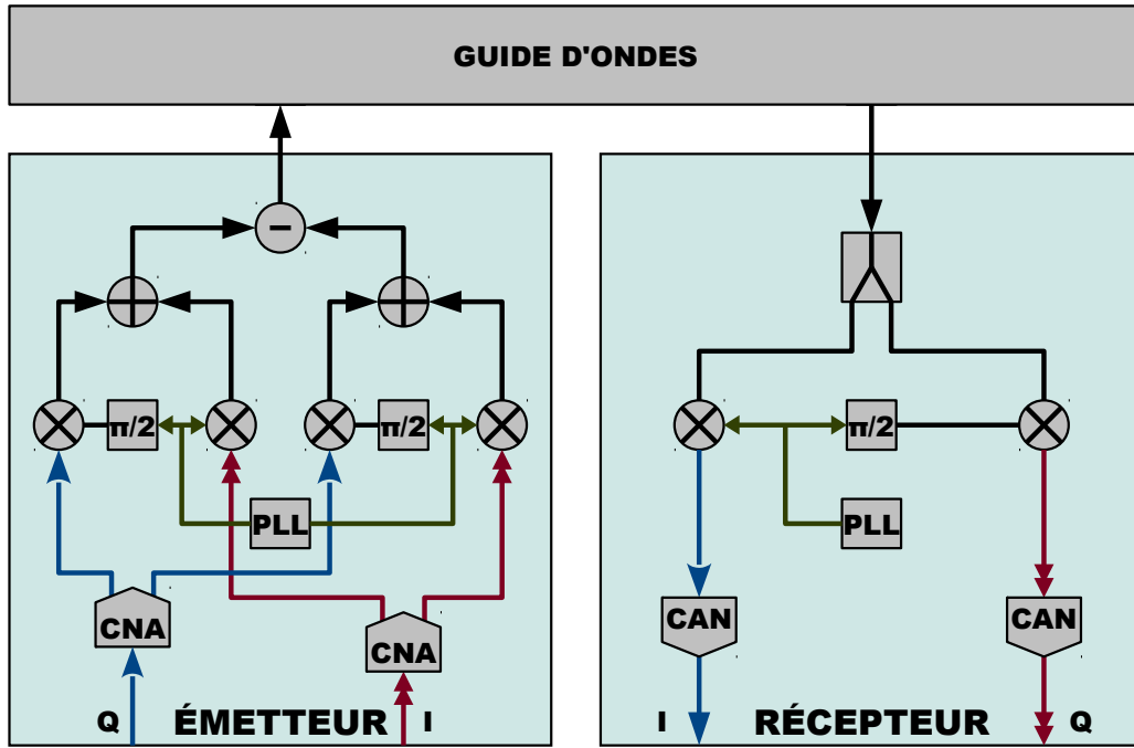
Figure 6.6 – Architecture des émetteurs et récepteurs de l'interface RF
