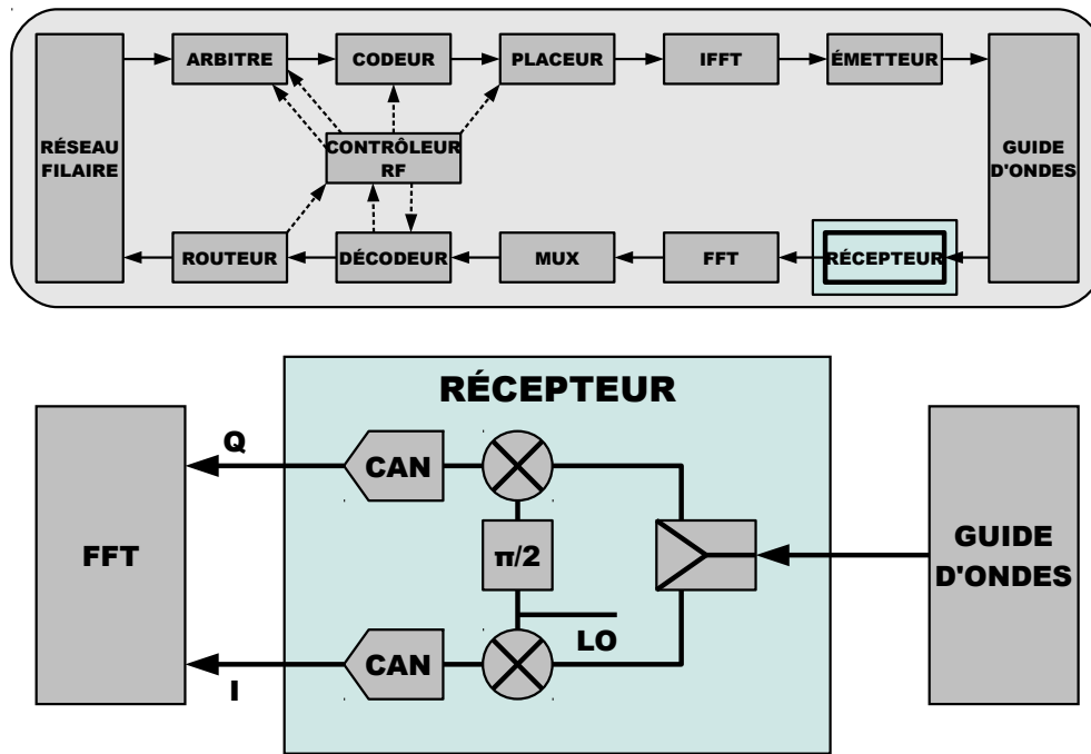
Figure 4.9 – Bloc de réception RF
