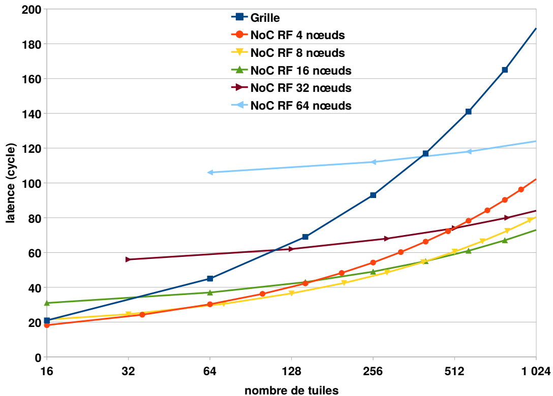
Figure 6.3 – Latence maximale du broadcast d'un FLIT sur une grille et sur un NoC RF ayant autant de canaux que de nœuds
