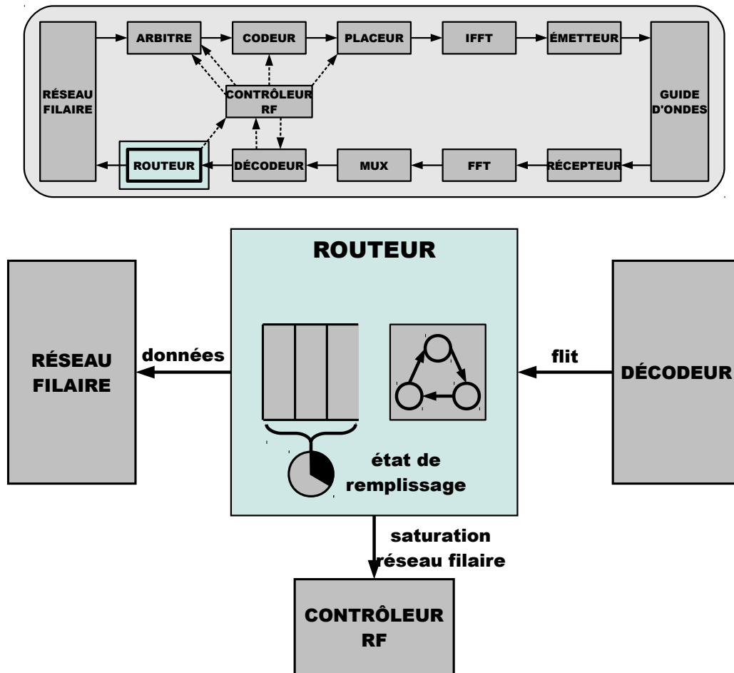
Figure 4.13 – Routeur
