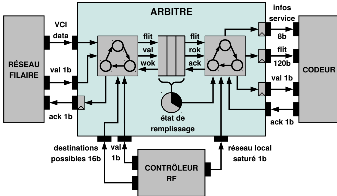
Figure 5.3 – Modèle de l'arbitre
