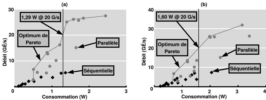
Figure 6.8 – Consommation (W) en fonction du taux d'échantillonnage (Giga Échantillons par seconde) de FFT 1024 (a) et 4096 (b) points pour une implémentation ASIC 65 nm ( extrait de [Milder et al., 2012] )
