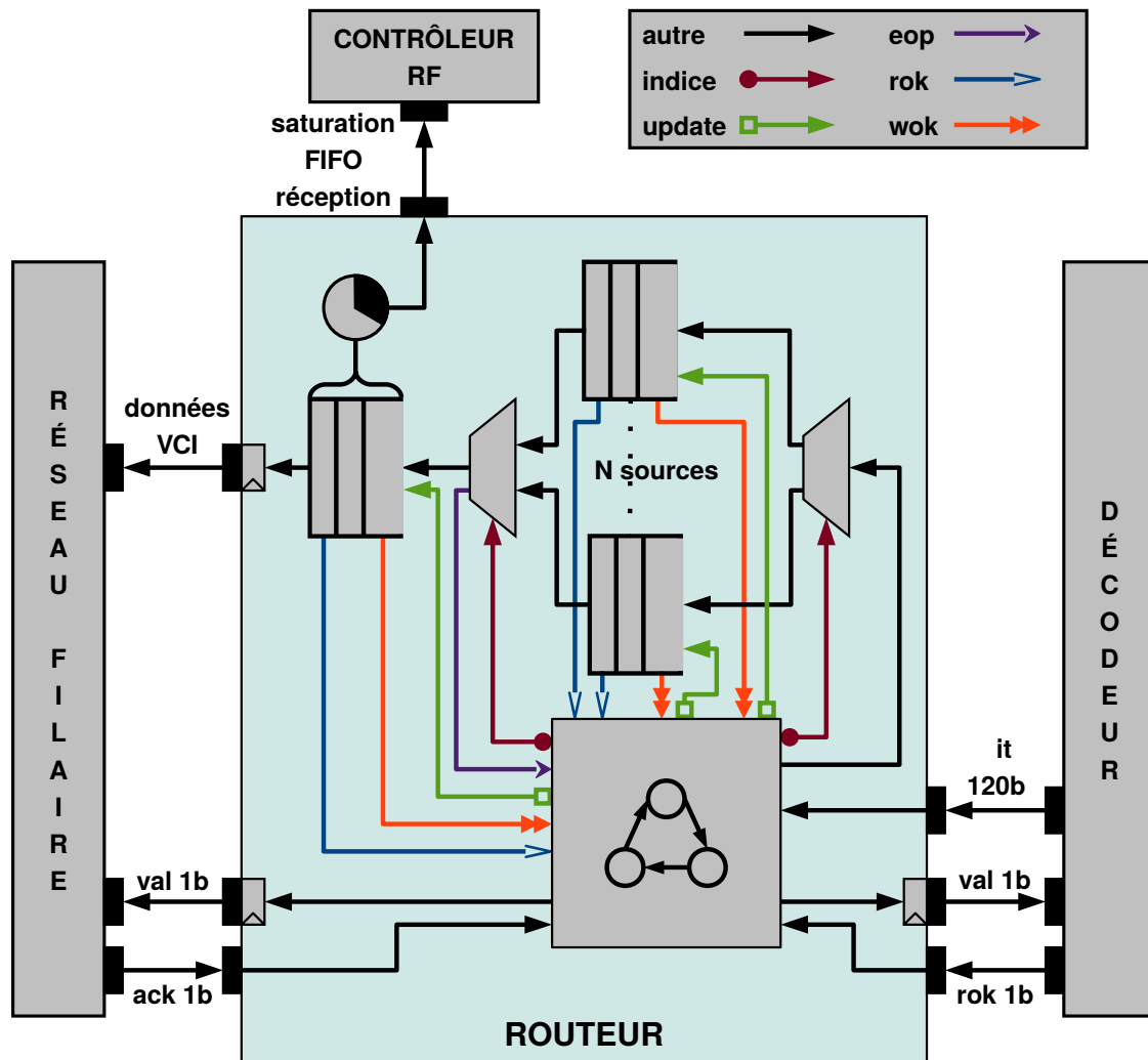
Figure 5.9 – Modèle du routeur
