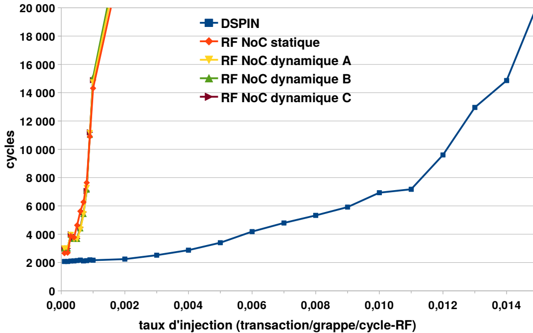
Figure 6.14 – Latence des communications de type broadcast avec réponse d'acquiescement pour un CMP 32 \times 32
