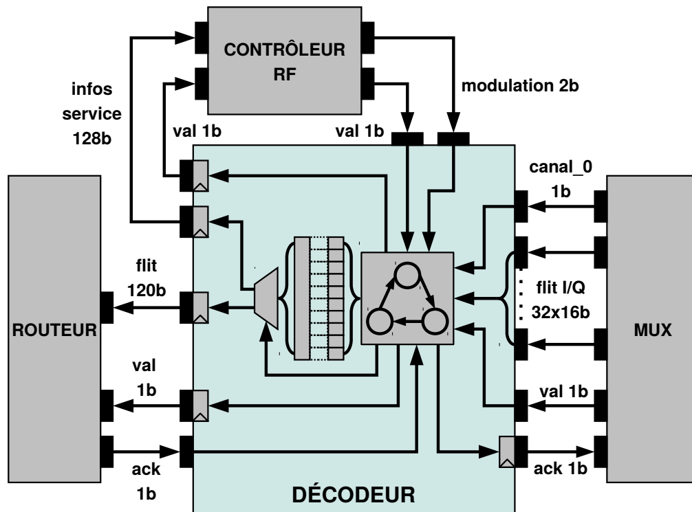
Figure 5.8 – Modèle du décodeur
