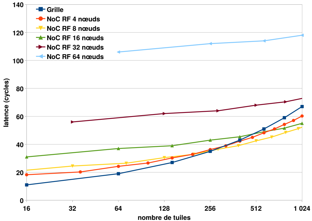
Figure 6.1 – Latence moyenne du transfert point à point d'un FLIT sur une grille et sur un NoC RF ayant autant de canaux que de nœuds
