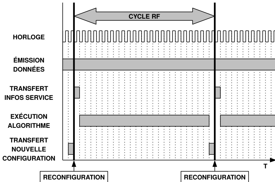
Figure 4.15 – Chronogramme du schéma d'allocation du contrôleur RF
