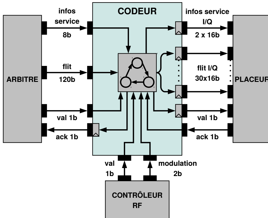
Figure 5.4 – Modèle du codeur
