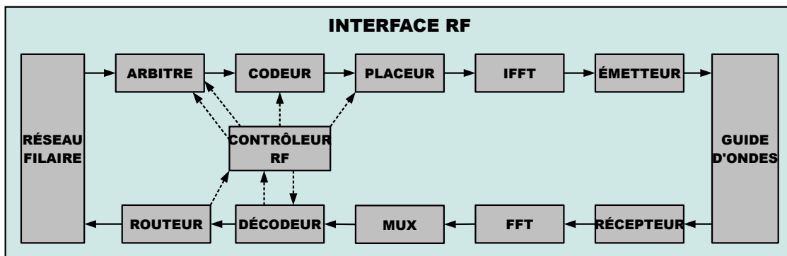
Figure 6.5 – Schéma bloc de l'Interface RF
