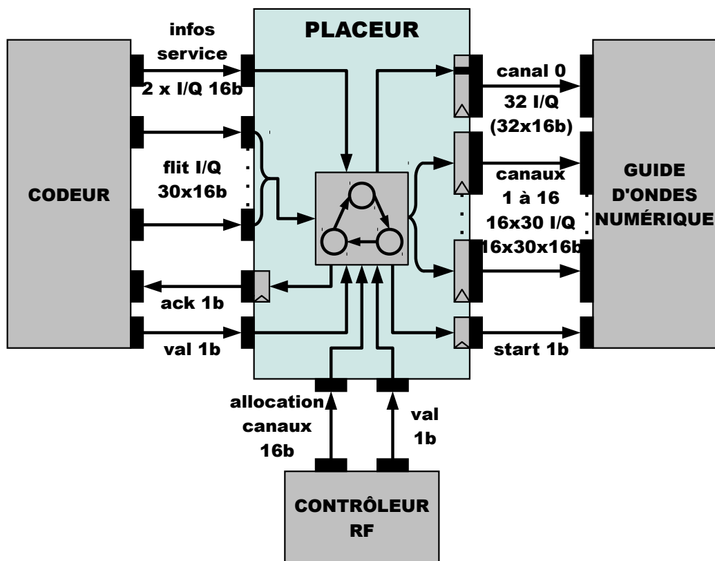
Figure 5.5 – Modèle du placeur
