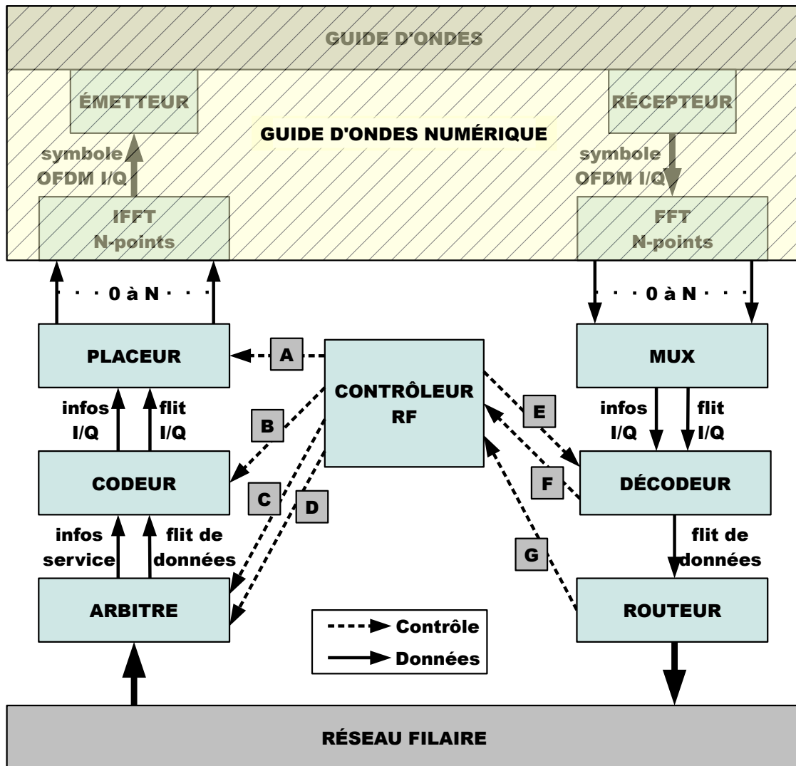
Figure 5.1 – Modèle de l'interface RF
