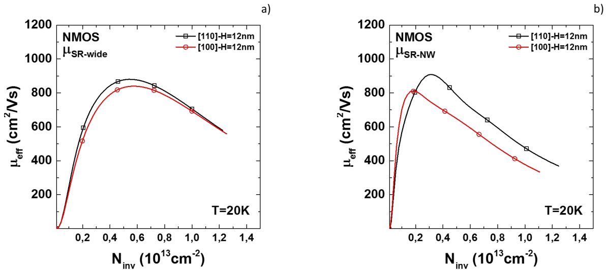
Figure 3.10.: Mobilité effective mesurée à T=20K en fonction de la densité de porteurs en inversion pour des transistors NMOS : (a) planaires ( W_{top} = 10\mu m , H = 12nm ), et (b) nanofils ( W_{top} = 20nm , H = 12nm ). Les deux orientations de canal \langle 100 \rangle et \langle 110 \rangle ont été mesurées.
