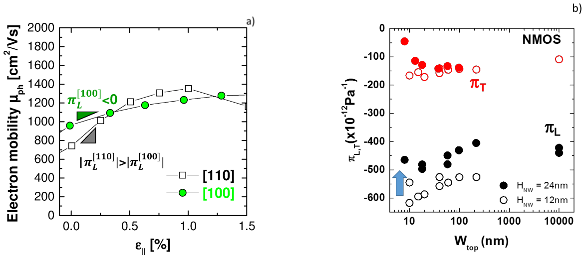
Figure 4.8.: a) Mobilité des électrons limitée par les phonons calculée en fonction d'une déformation uniaxiale \epsilon_{||} parallèle au transport dans un nanofil ( d=8 nm, d'après [81]). b) Évolution du coefficient piézorésistif avec la largeur des nanofils pour deux hauteurs de canal différentes H_{NW}=12 nm et H_{NW}=24 nm ( L_G = 10\mu m , N_{inv} = 0.8 \times 10^{13} cm^{-2} ).
