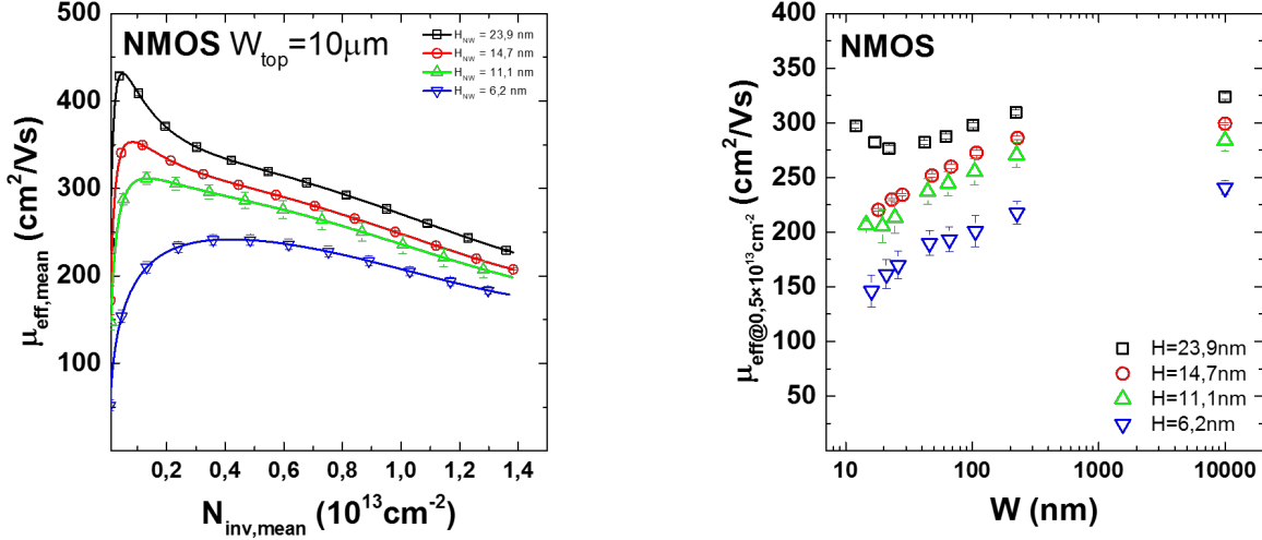
Figure 3.5.: a) Mobilité effective en fonction de la charge d'inversion mesurée pour des transistors NMOS planaires ( W_{NW} = 10 \mu\text{m} ) et pour différentes épaisseurs de canal H_{NW} = [24 - 6] \text{nm} . b) Mobilité effective à N_{\text{inv}} = 0.5 \cdot 10^{13} \text{cm}^{-2} en fonction de la largeur w_{\text{top}} et de l'épaisseur du canal H .
