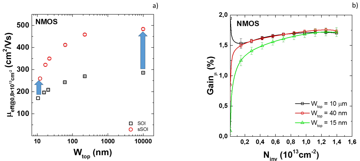
Figure 4.9.: a) Évolution de la mobilité effective avec la largeur des nanofils pour des dispositifs NMOS sSOI (ronds rouges - 1.4GPa) et SOI (carrés noirs - 0 GPa) ( L_G = 10\mu\text{m} , N_{\text{inv}} = 0.8 \times 10^{13} \text{ cm}^{-2} ). b) Gain de mobilité en fonction de la densité de porteurs en inversion N_{\text{inv}} pour trois largeurs de grille : noir dispositifs planaires W_{\text{top}} = 10\mu\text{m} , rouge dispositifs nanofils intermédiaires W_{\text{top}} = 40\text{nm} et nanofils W_{\text{top}} = 10\text{nm}
