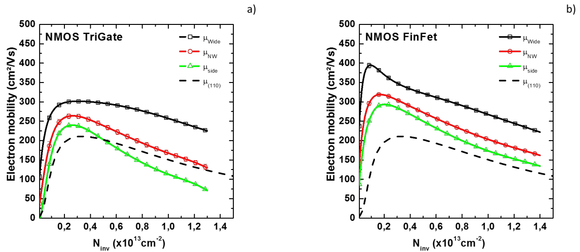
Figure 3.24.: Mobilité mesurée pour des dispositifs NMOS TriGate H_{NW} = 12nm (a) et FinFet H_{NW} = 24nm (b) en fonction de la densité de porteurs en inversion. Dispositifs planaires : ligne noire, dispositifs nanofils : ligne rouge, mobilité des surfaces latérales calculées avec l'équation 3.23 : ligne verte, mobilité universelle pour une surface d'inversion (110) ligne noire pointillée.
