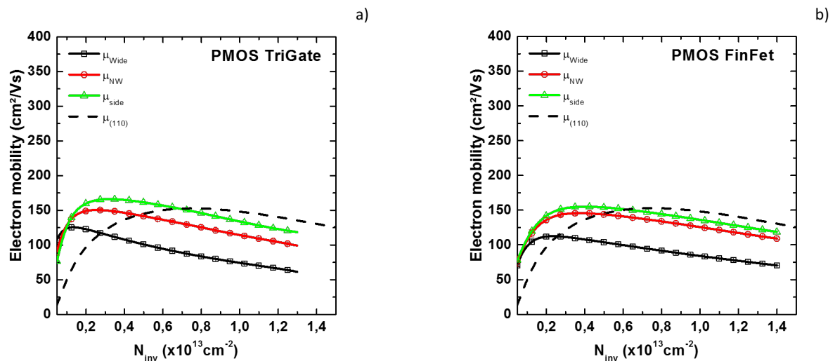
Figure 3.25.: Mobilité mesurée pour des dispositifs PMOS TriGate H_{NW} = 12nm (a) et FinFet H_{NW} = 24nm (b) en fonction de la densité de porteurs en inversion. Dispositifs planaires : ligne noire, dispositifs nanofils ( W_{top}=12nm ) : ligne rouge, mobilité des surfaces latérales calculées avec l'équation 3.23 : ligne verte, mobilité universelle pour une surface d'inversion (110) ligne noire pointillée.
