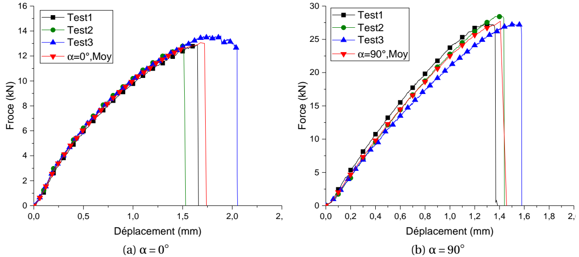
FIGURE 4.18 – Résultats expérimentaux des chargements purs en configuration (1-3)
