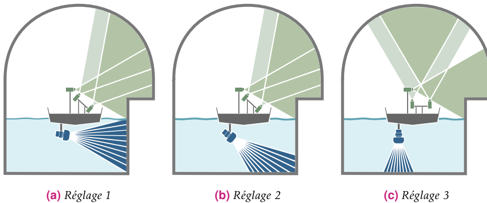
FIGURE 3.6 – Vue schématique des trois configurations (3 angles de sonar et 2 angles du capteur stéréo) utilisées pour numériser un demi-tunnel.
