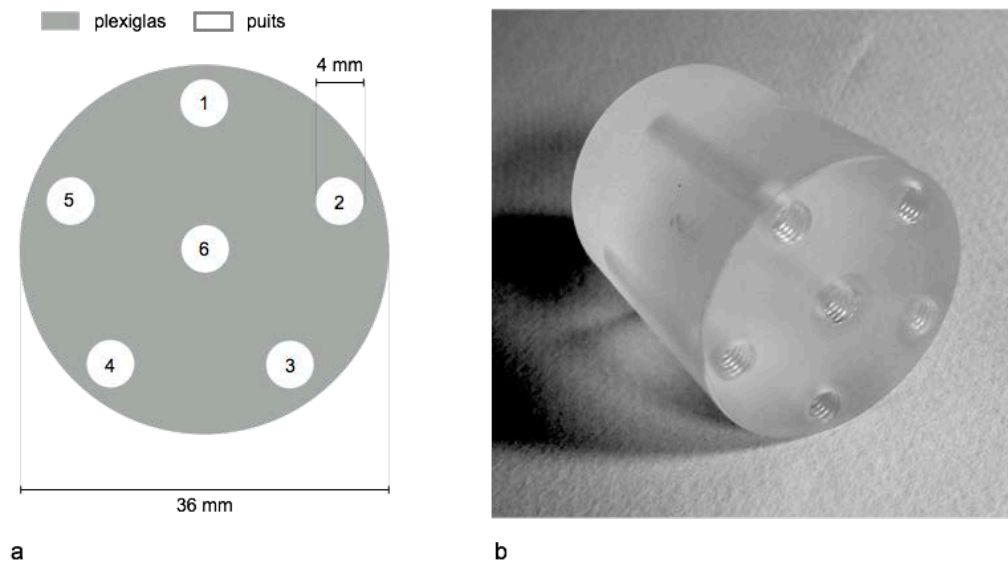
Figure 2.29 - Plan axial (a) et photographie (b) du module de linéarité.
