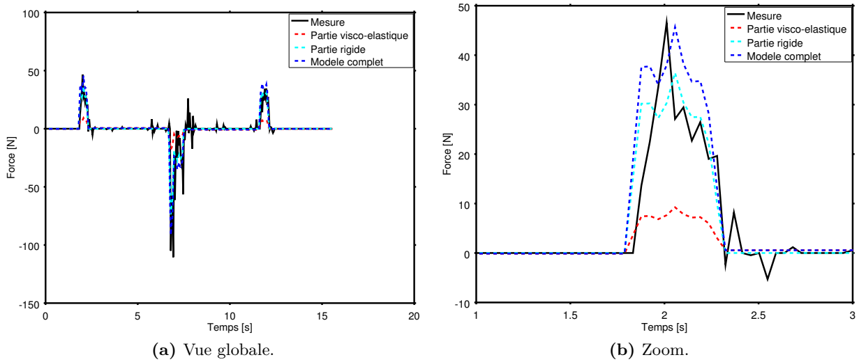
Figure 5.27 – Force prédite par un modèle en masse purement inertielle, la partie visco-elastique du modèle Kelvin-Voigt ainsi que le modèle Kelvin-Voigt dans son ensemble pour un volontaire de 82 kg et 1,72 m.
