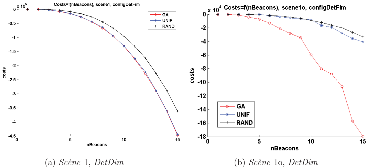
FIGURE 5.9 – coût = f(nBalises) pour la fonction de coût DetDim et les Scènes 1 et 1o
