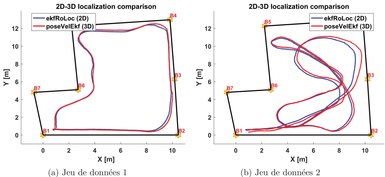
FIGURE 3.27 – Comparaison des trajectoires estimées par les filtres EKF 2D et 3D pour deux jeux de données réalisés avec le prototype
