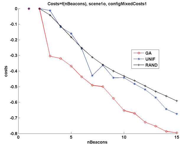
(b) Scène 1o, MixedCosts1
