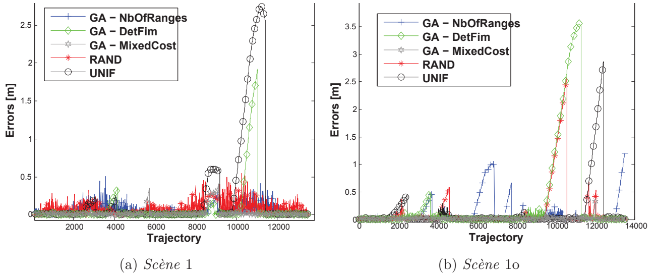
FIGURE 5.14 – Évolution des erreurs de la localisation pour les Scène 1 (a) et Scène 1o (b). Les pics correspondent à des zones du terrain où l'estimation de la position par trilatération n'est pas possible à cause d'un nombre insuffisant de balises pour effectuer le calcul.
