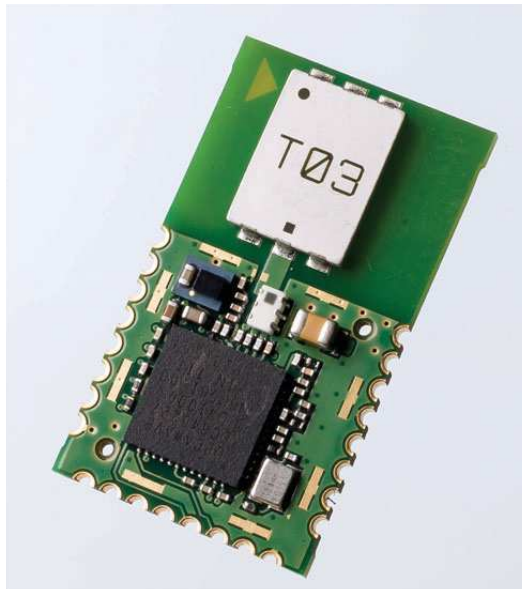
FIGURE 2.7 – Module DWM1000 de Decawave ( http://www.decawave.com ) utilisé pour obtenir les mesures de distance
