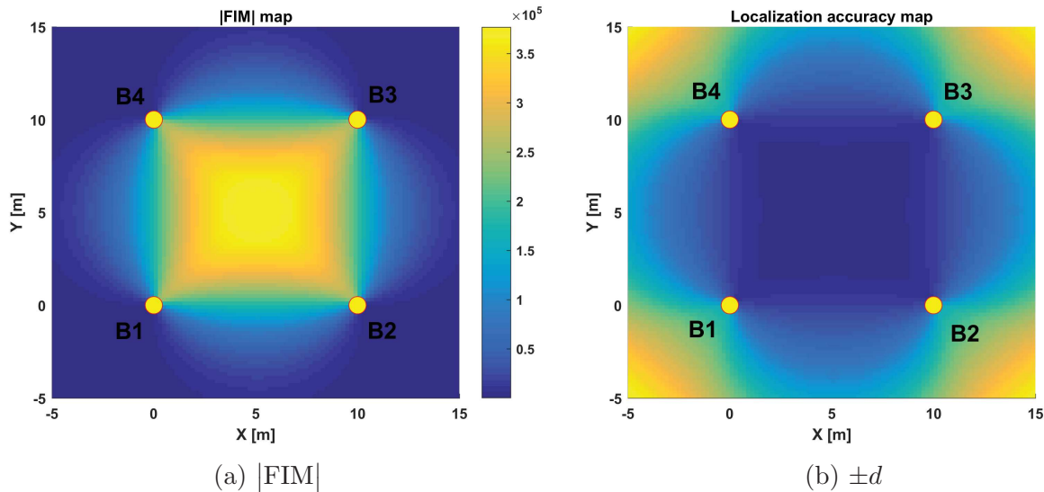
FIGURE 5.5 – Valeurs de |FIM| (a) et précision de localisation (b) dans le cas d'un placement de 4 balises
