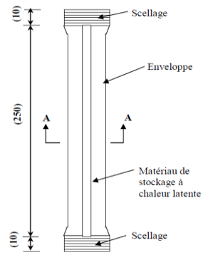
Figure 2- Brique de MCP ECOJOULE 108.
