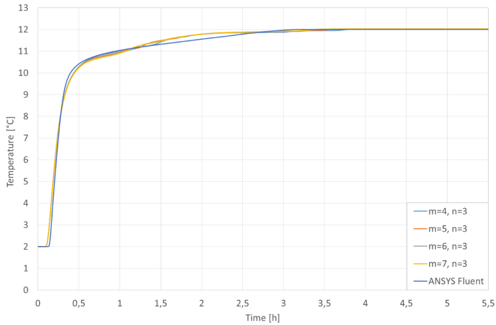
Figure 13 - Valeurs de la température en fonction du temps pour le nœud ( i = w, j = n ) et pour son équivalent dans le modèle ANSYS Fluent pendant la phase de décharge du système.
