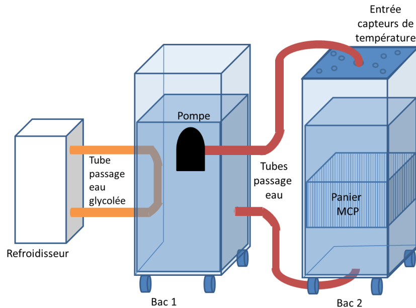
Figure 16: Schéma du prototype expérimental.
