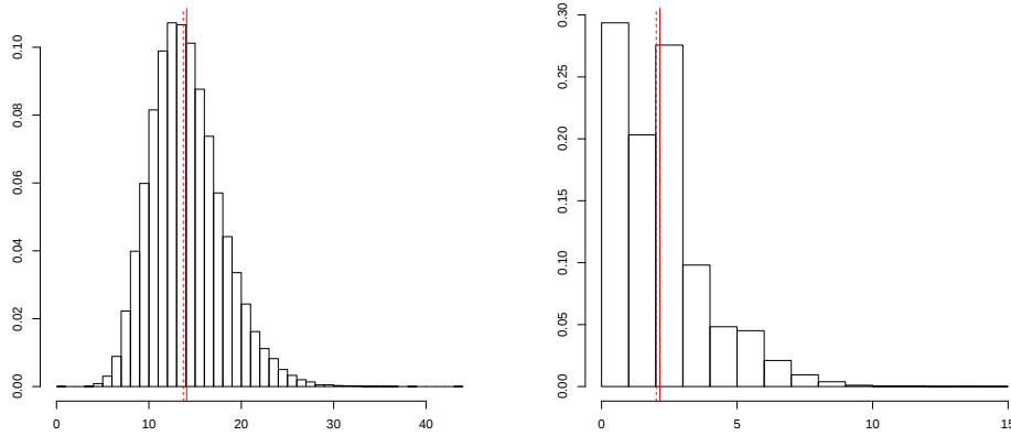
Figure 3.16: Distribution a posteriori de \frac{1}{2\sigma^2}SCR et de \tau \times \text{dist}^2(\beta^s, \bar{\beta}_E^s; \bar{g}_E) pour les données de Pernes-Les-Fontaines ( \tau fixé par validation croisée bayésienne). Le premier (resp. second) graphique est un histogramme des valeurs de \frac{1}{2\sigma^2}SCR (resp. de \tau \times \text{dist}^2(\beta^s, \bar{\beta}_E^s; \bar{g}_E) ) calculé à partir de l'échantillon MCMC. Pour ces deux graphiques, la droite rouge en trait plein (resp. en pointillé) correspond à la moyenne (resp. médiane) de la distribution représentée.
