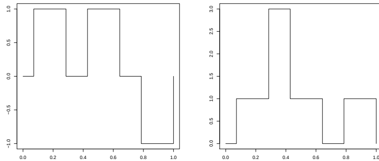
Figure 3.3: Représentation de la connaissance des experts (simulés) en utilisant la procédure d'éllicitation décrite en section 3.3. Le premier (resp. second) graphique donne la fonction \bar{\beta}_E^s (resp. \bar{g}_E ), la fonction signe moyenne des experts (resp. la certitude totale des experts).
