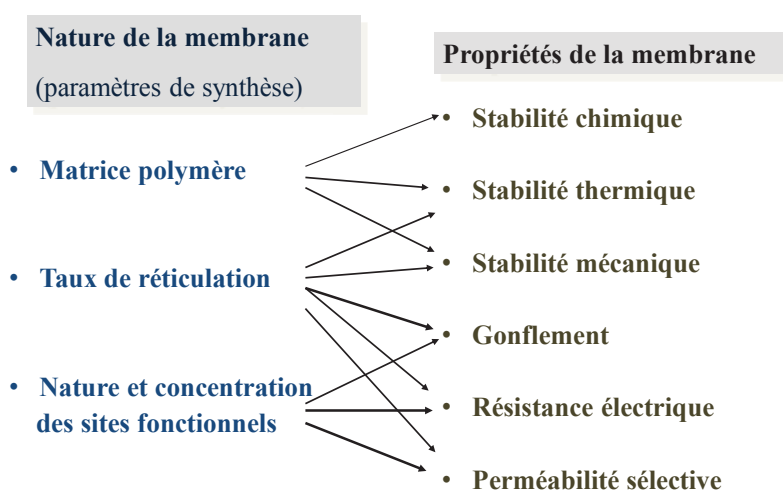
Figure 1.3 – Relations entre les paramètres de synthèse et les propriétés d'une MEI
