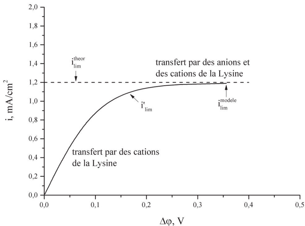
Figure 4.27 – Système \text{LysHCl}/\text{Nafton} : Courbe courant tension calculée
