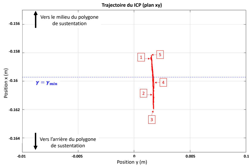
FIGURE 6.9 – Équilibre de l'exosquelette dans le plan sagittal - Position du point de capture instantané dans le plan transversal (x;y). Les numéros indiqués représentent les différentes étapes mentionnées ci-dessus.
