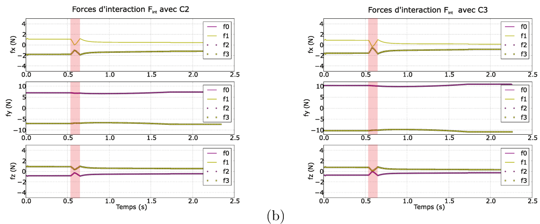
FIGURE 5.10 – [139]. Forces d’interaction entre l’utilisateur et l’exosquelette via les points d’interaction choisis (cf. figure (5.9)) issues du calcul d’optimisation des couples articulaires : - (a) avec le critère C_2 - (b) avec le critère C_3 .
