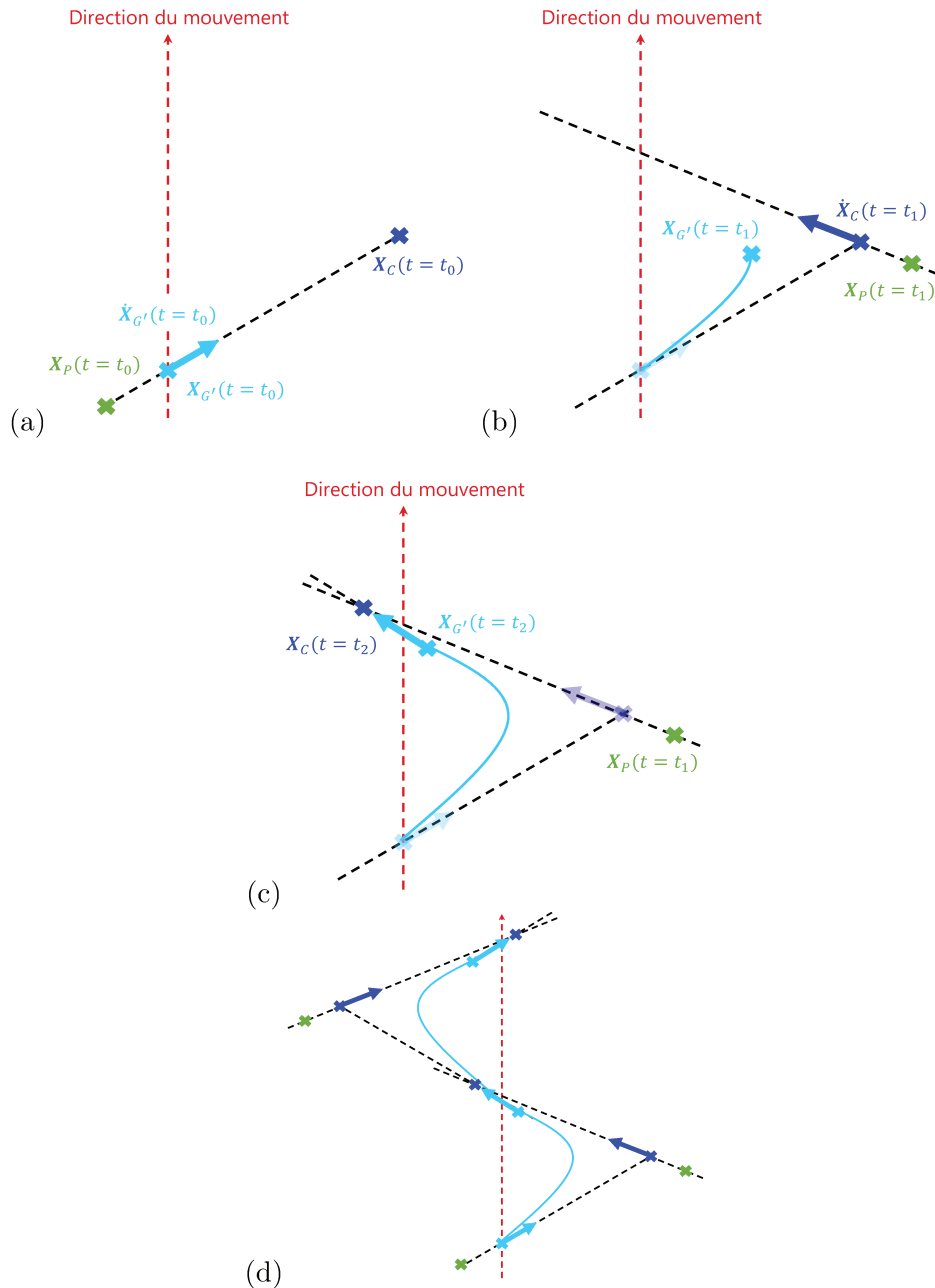
FIGURE 3.1 – Schéma illustrant la génération d'une trajectoire du GCOM à partir d'une commande basée sur le ICP. (a) A t = t_0 , G' a une vitesse \dot{X}_{G'} , on calcule la position du ICP (eq. (2.5.1)). Si la position de P n'est pas modifiée, G' reste sur la même ligne. (b) A t = t_1 , pour modifier la trajectoire du GCOM, il faut changer la direction de \dot{X}_C en plaçant judicieusement P (eq. (3.3)). (c) G' converge naturellement vers C (eq. (3.2)). (d) Exemple de trajectoire pour G' .
