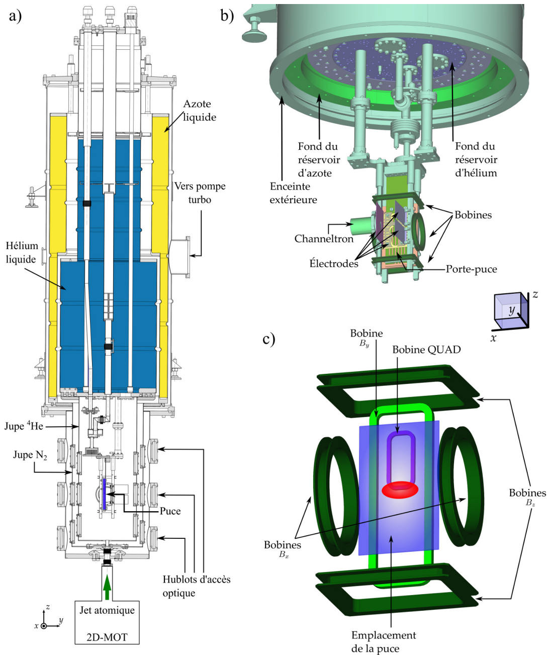
Figure II.1 Schéma du dispositif cryogénique : a) Coupe du du cryostat, avec la puce (colorée en violet) tournée vers le côté droit. Le réservoir d'azote liquide est indiqué en jaune, le réservoir d'hélium liquide en bleu. Le cœur de l'expérience est visible, ainsi que les deux « jupes » et l'enceinte extérieure à température ambiante. Cinq hublots, trois en face de la puce et un sur chaque côté, sont installés sur chacune de ces jupes pour l'accès optique. Derrière la puce, du côté gauche du schéma, les hublots optiques sont remplacés par des disques métalliques. Les atomes proviennent du « 2D-MOT », une enceinte externe située sous le cryostat, où l'on réalise un piège magnéto-optique à deux dimensions. b) Vue schématique du cœur de l'expérience. La puce est fixée sur le porte-puce et fait face à la direction y . Les bobines (vert foncé) servent à créer des champs magnétiques pour le piégeage des atomes de rubidium. Le channeltron et les différentes électrodes représentées servent à la détection des atomes de Rydberg. On ne voit pas les « jupes » d'azote et d'hélium, ni l'enceinte extérieure. c) Vue de près des bobines : la bobine QUAD (mauve) génère un champ quadrupolaire pour faire un MOT sur puce. L'emplacement de la puce est représenté par le rectangle bleu devant la bobine QUAD et la bobine B_y (vert clair). La zone rouge indique l'endroit où les atomes de rubidium sont piégés, devant la puce. Les axes sont les mêmes qu'en b) .
