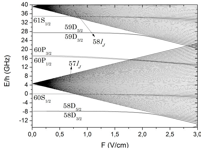
Figure I.2 Diagramme Stark autour du niveau 60S , pour les états de m_j = 1/2 . Le défaut quantique déplace beaucoup les niveaux S,P et D. Ces niveaux non-dégénérés ont un effet Stark quadratique en champ électrique. Les niveaux de grand l sont dégénérés et ont un effet Stark linéaire (ce sont les multiplicités qui s'ouvrent en éventail).
