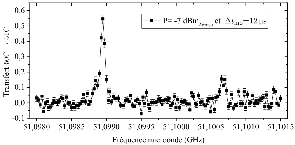
Figure V.25 Spectre microonde 50C-51C optimisé. Le pic principal centre en 51,0989 GHz correspond à la transition 50C \rightarrow 51C. Un ajustement lorentzien donne une largeur spectrale est de 67,5 kHz. Le petit pic centré en 51,1007 GHz correspond au transfert vers le niveau 51E + des quelques atomes que le passage adiabatique a amené dans le niveau 50E + .
