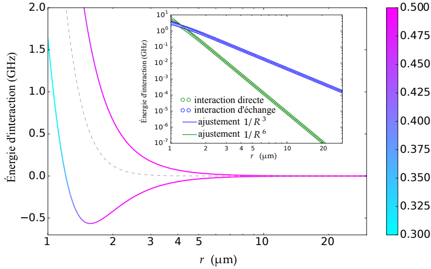
Figure I.13 Énergie de la paire 60S-60P 3/2 en présence de l'interaction dipolaire. Les branches inférieure et supérieure correspondent respectivement aux superpositions symétrique et antisymétrique des deux niveaux de départ. L'échelle de couleur représente le carré de la projection sur l'état non perturbé |60S, 60P_{3/2}\rangle . La ligne pointillée représente le déplacement en énergie dû à l'interaction directe. L'insert représente le déplacement d'énergie ainsi que le terme d'échange en échelle log-log et leurs ajustements en 1/r^6 et 1/r^3 respectivement.
