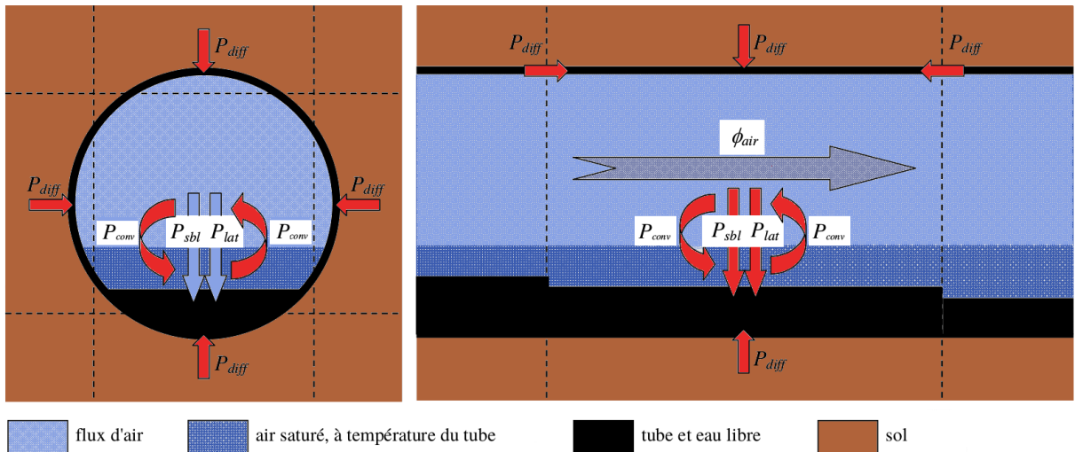
Figure 2.7 – Schématisation des échanges sensibles P_{sbl} , latents P_{lat} , diffusifs P_{diff} et convectifs P_{conv} au niveau du segment du tube [Hol02].
