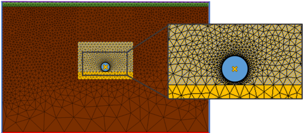
Figure 5.5 – Représentation du maillage du modèle numérique 2D.
