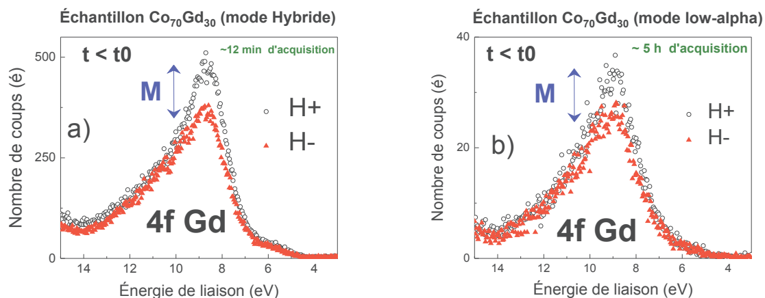
Figure I.9 : Nombre de photoélectrons en fonction de leur énergie cinétique au seuil Gd M_5 pour deux polarisations magnétiques différentes dans l'alliage \text{Co}_{70}\text{Gd}_{30} avant l'impulsion laser a) en mode hybride (12 min d'acquisition) et b) en mode low-alpha (5 h d'acquisition).
