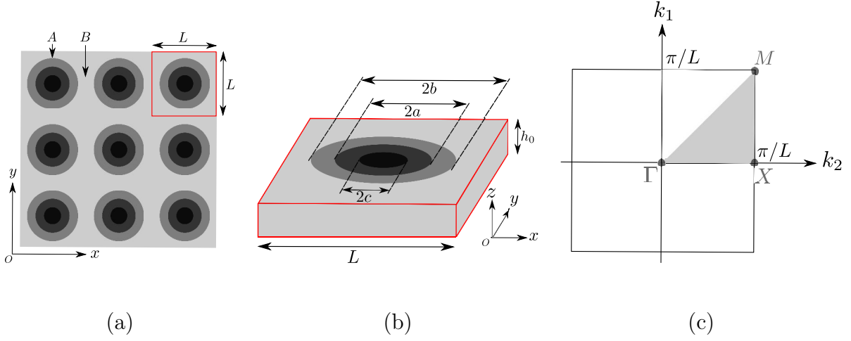
FIGURE 4.9 – (a) : Schéma illustrant la vue de dessus de la méta-plaque étudiée. (b) : Cellule unitaire carrée. (c) : Première zone de Brillouin de la cellule unitaire, où le triangle grisé, délimité par \Gamma XM , représente la zone de Brillouin irréductible.
