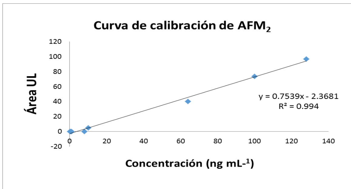
Figura. A4.2. Curva de calibración AFM 2 .
