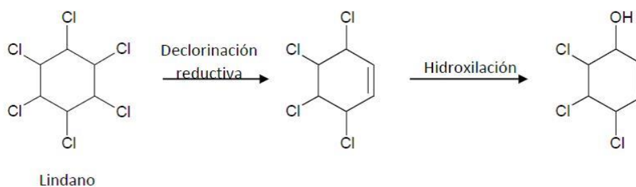
Figura 2.6 Reacción de degradación de lindano por hongos de pudrición blanca (Singh et al. , 1999).
