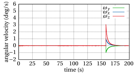
(d) Angular velocities
