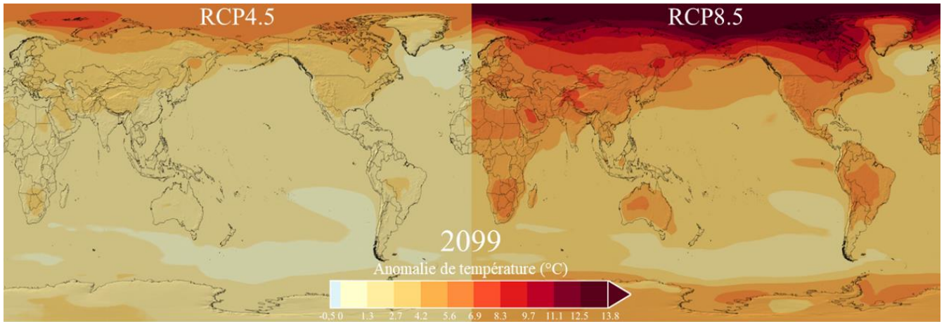
Figure 1. Prédiction des anomalies de température à la surface du globe pour 2099. Les données proviennent d'une moyenne des prédictions des modèles du CMIP5 (Coupled Model Intercomparison Project Phase 5). Source : NASA Center for Climate Simulation/Scientific Visualization Studio.
