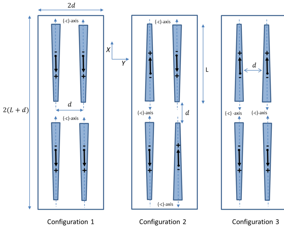
Figure 50. Trois configurations de réseaux bidimensionnels de fils étudiées. Les schémas montrent la position relative des fils vis-à-vis de l'axe de croissance ( \vec{c} ) ainsi que les dimensions.
