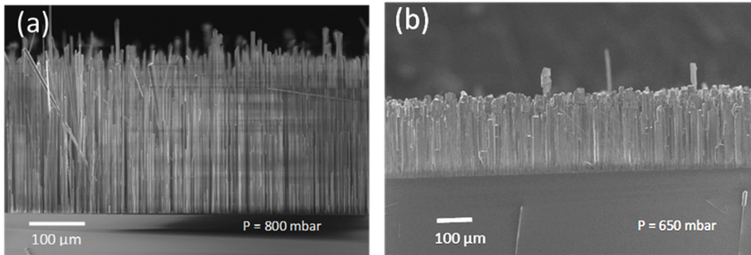
Figure 21. Images MEB de fils de GaN obtenus en MOVPE avec des conditions de pression de (a) 800 mbar et (b) 650 mbar.
