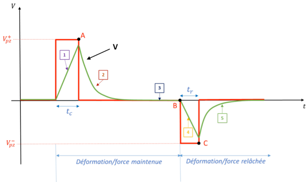
Figure 105. Schéma agrandi du processus de génération de la tension piézoélectrique en analogie avec le modèle électrique.
