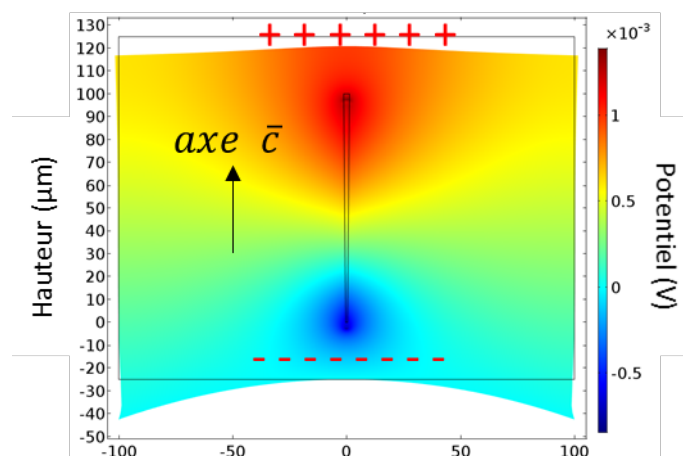
Figure 80. Cartographie du potentiel électrique au sein d'une couche de PDMS contenant un fil unique de 100 \mu\text{m} de longueur soumise à une flexion de 10 cm de rayon de courbure appliquée au niveau de la face inférieure. La masse est définie au niveau de cette même face.
