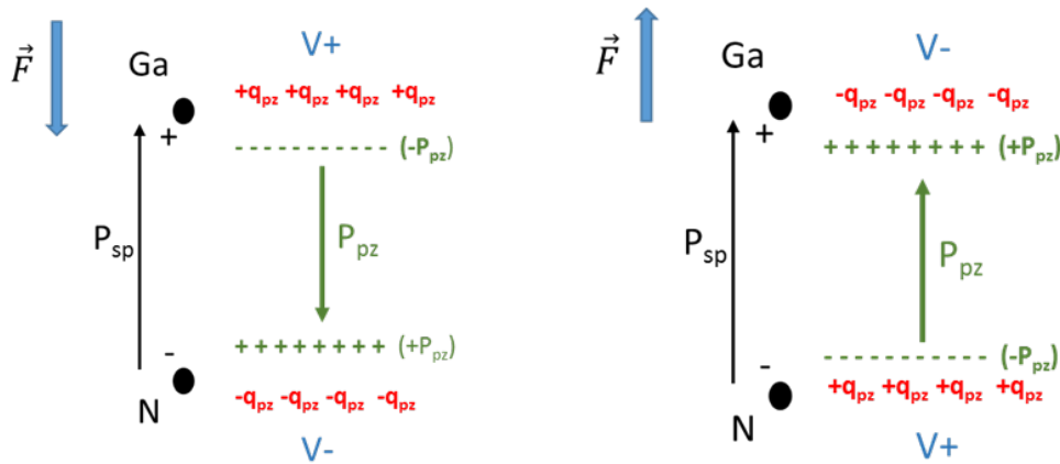
Figure 10. Représentation schématique de la distribution des charges piézoélectriques, des champs électrique et de polarisation sous compression et élongation pour un cristal de GaN de polarité N.
