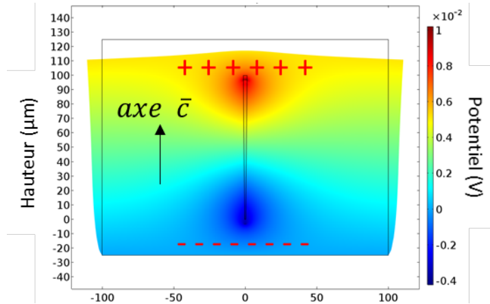
Figure 79. Cartographie du potentiel électrique au sein d'une couche de PDMS contenant un unique fil de GaN de 100 \mu\text{m} de longueur, soumise à une compression de 5 \text{ nN}/\mu\text{m}^2 uniformément appliquée sur la face supérieure. La masse est définie au niveau de la face inférieure.
