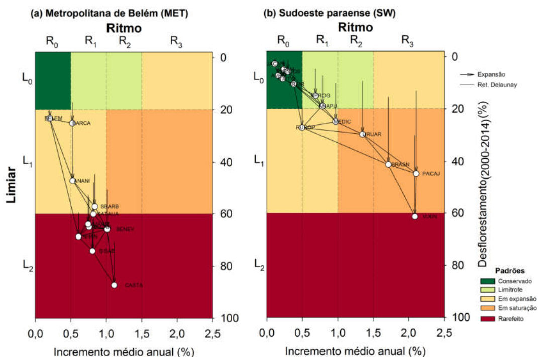
Figura C-6 Disposição da extensão das taxas e ritmo de desflorestamento dos municípios nas mesorregiões (a) MET e (b) SW do estado do Pará, em função das tipificações propostas, agregadas sob reticulação do tipo Delanauy
