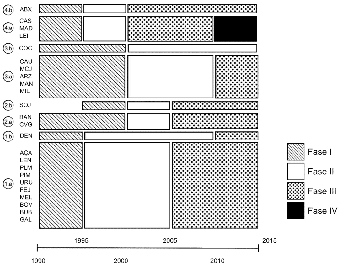
Figura A-74 Disposição das fases das cadeias agropecuárias e extrativistas, ao longo da série histórica (1990-2014) (IBGE, 2016)
