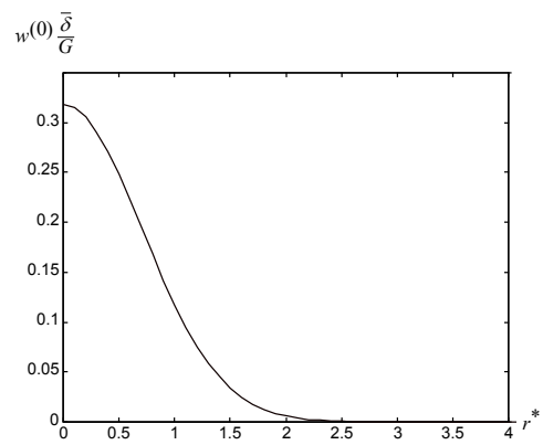
Figure 3.3 w^{(0)}\frac{\bar{\delta}}{G} en fonction de r^*
