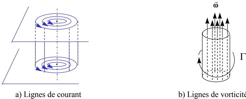
Figure 3 : Sch  ma d'une tornade
