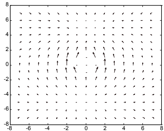
Figure 3.15 Champ \left(\frac{u_{so}^{(1)}}{K^{(0)}}, \frac{v_{so}^{(1)} + v_r^{(1)}}{K^{(0)}}\right) dans le plan (r^*, \varphi) pour G=1
