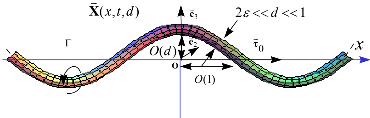
Figure 6.8 Le filament droit et sa perturbation
