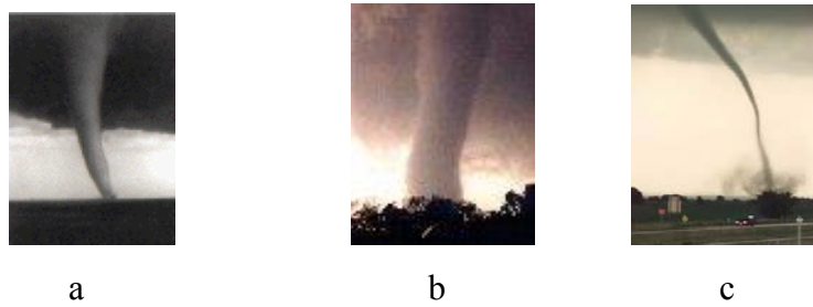
Figure 4 : Photographies de tornades
