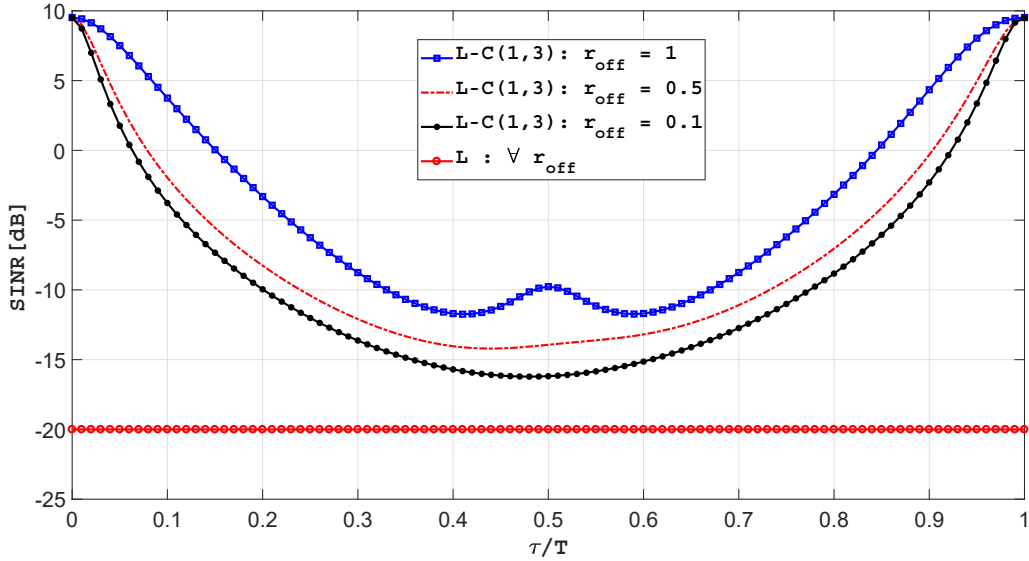
FIGURE 3.12 – \text{SINR}_{\text{LC}(1,3)} comparé au \text{SINR}_L pour des symboles SOI et CCI QPSK en fonction de \tau/T pour \phi = 0 , \text{SNR} = 10\text{dB} et \text{INR} = 30\text{dB} .
