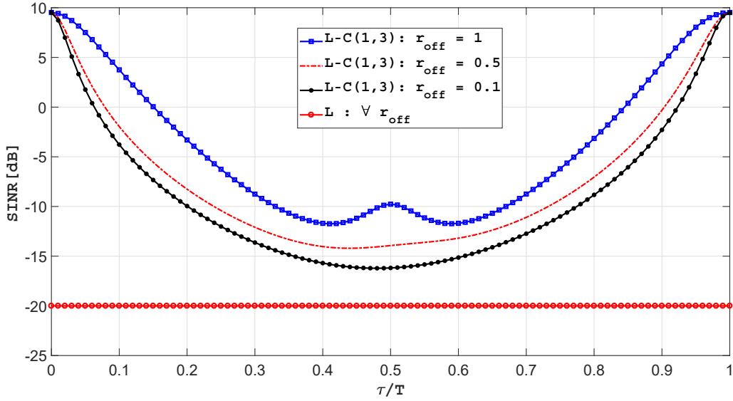
FIGURE 3.12 – \text{SINR}_{\text{LC}(1,3)} comparé au \text{SINR}_{\text{L}} pour des symboles SOI et CCI QPSK en fonction de \tau/T pour \phi = 0 , \text{SNR} = 10\text{dB} et \text{INR} = 30\text{dB} .
