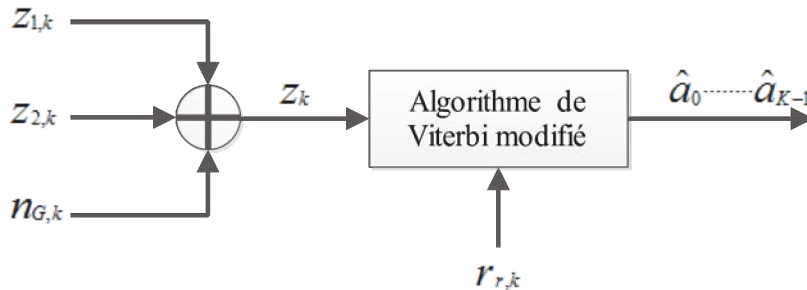
FIGURE A.16 – Modèle discret équivalent au récepteur SIMO MLSE de la figure A.15
