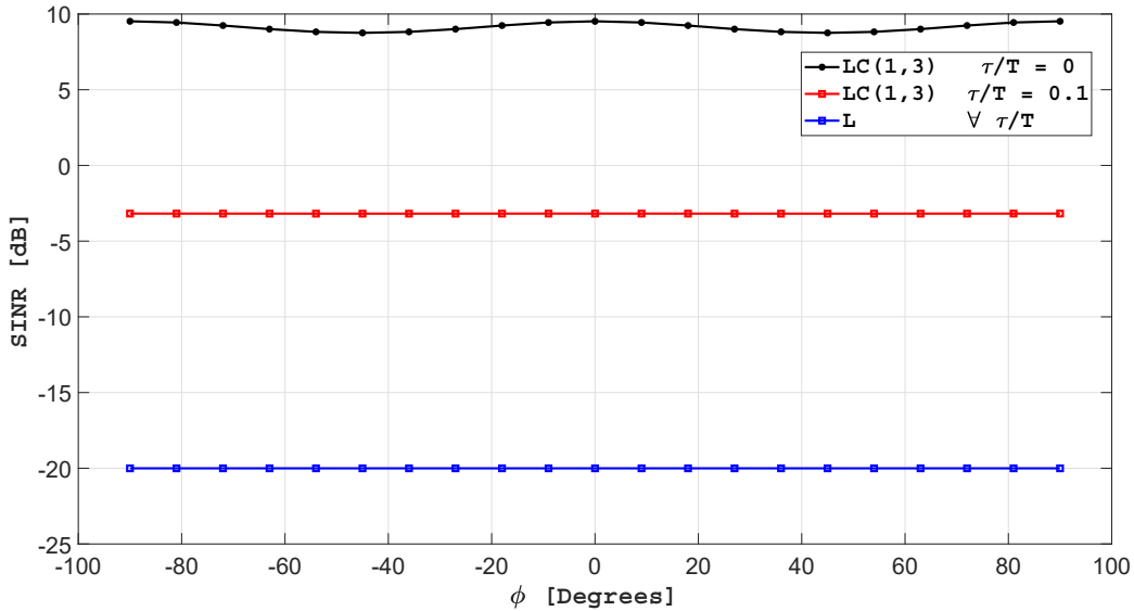
FIGURE 3.13 – \text{SINR}_{\text{LC}(1,3)} comparé au \text{SINR}_L pour des symboles SOI et CCI QPSK en fonction de \phi pour \text{SNR} = 10\text{dB} et \text{INR} = 30\text{dB} .
