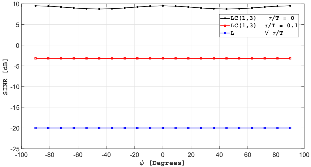
FIGURE 3.13 – \text{SINR}_{\text{LC}(1,3)} comparé au \text{SINR}_{\text{L}} pour des symboles SOI et CCI QPSK en fonction de \phi pour \text{SNR} = 10\text{dB} et \text{INR} = 30\text{dB} .
