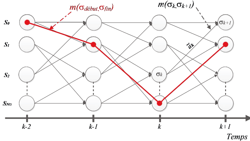
FIGURE A.28 – Treillis à N_\sigma = (\text{card}\mathcal{A})^{L_i} états pour la détection au sens ML d'un signal modulée linéairement à deux états ( \text{card}\mathcal{A} = 2 ) 6 et transmis à travers un canal sélectif en fréquence (étendue du canal discret équivalent = L_i + 1 ).
