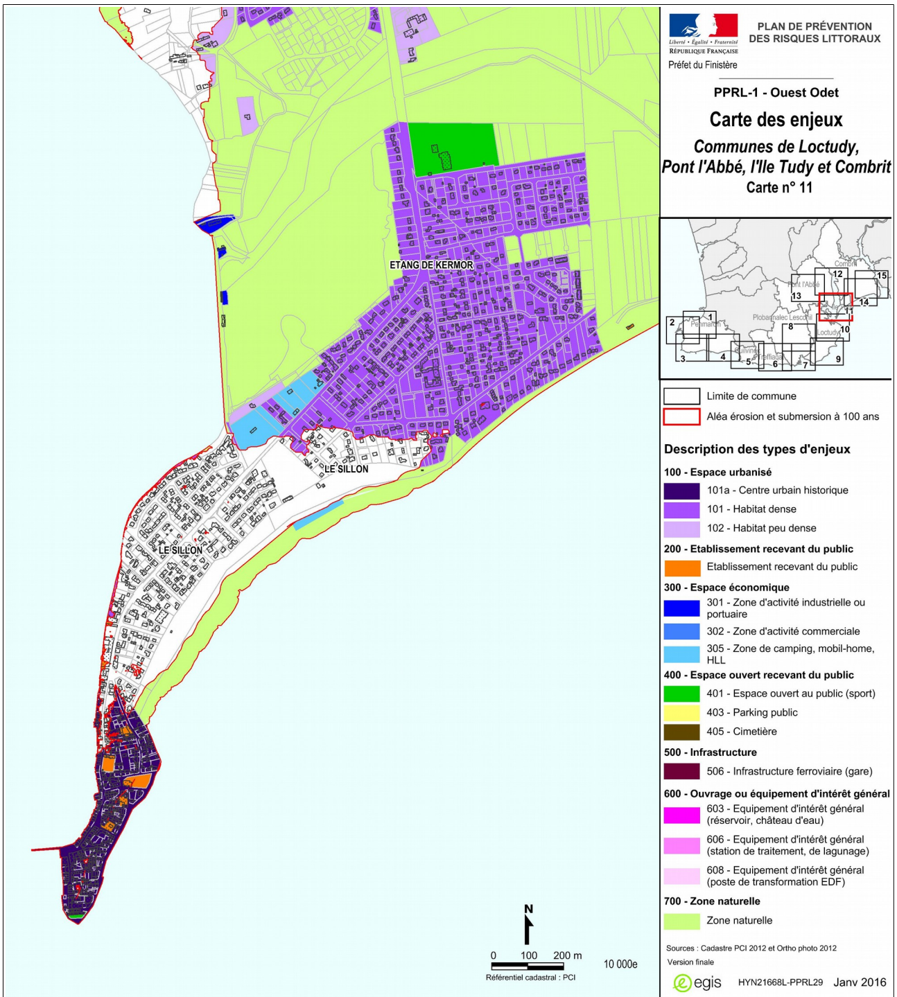
Figure 3. Carte des enjeux du PPRL de la commune de l'Ile-Tudy (29) (Préfecture du Finistère, PPRL Ouest Odet approuvé en 2016)
