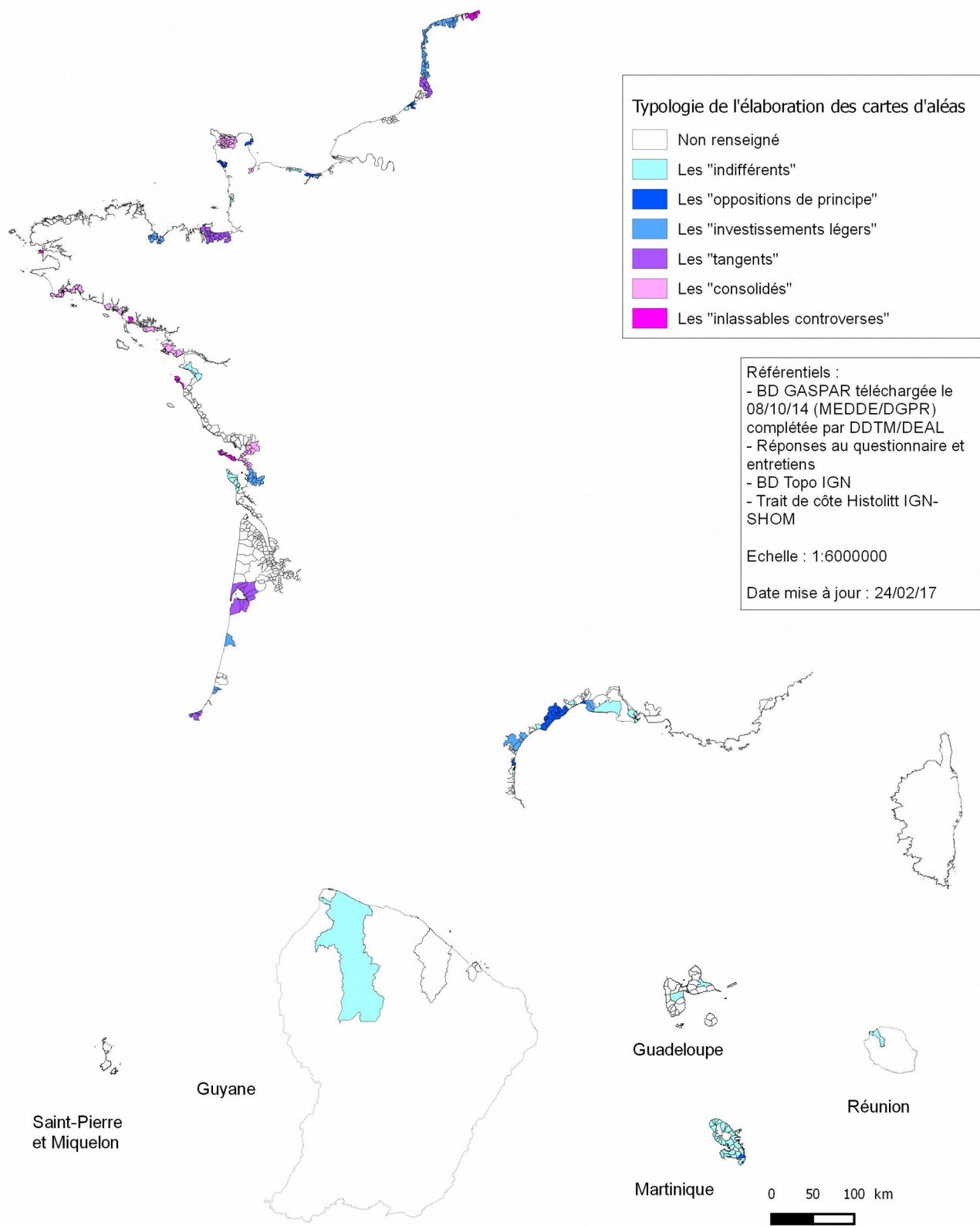
Figure 28. Carte des catégories de la typologie des démarches de concertation lors de l'élaboration des cartes d'aléas littoraux
