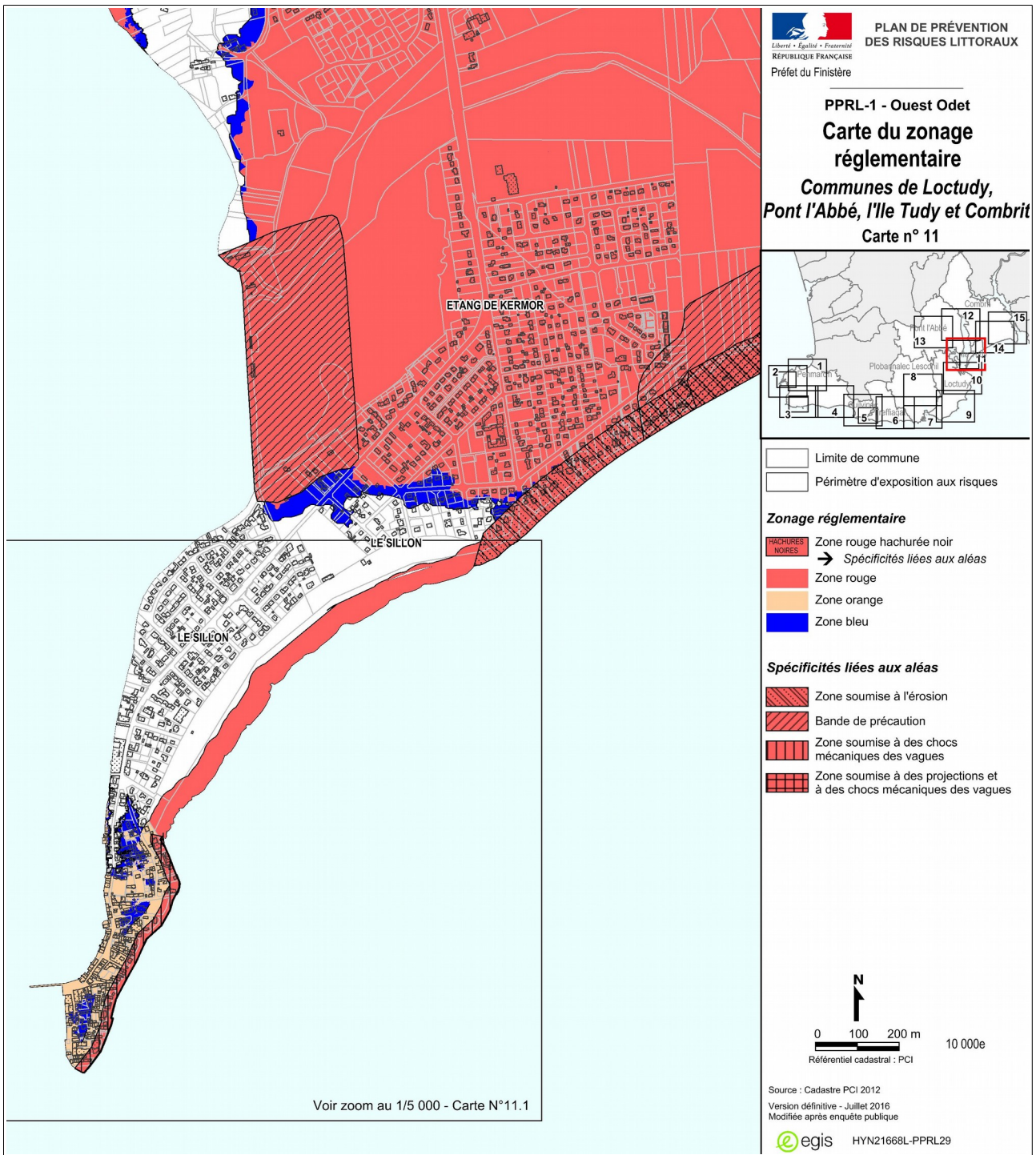
Figure 4. Carte du zonage réglementaire du PPRL de la commune de l'île-Tudy (29) (Préfecture du Finistère, PPRL Ouest Odet approuvé en 2016)
