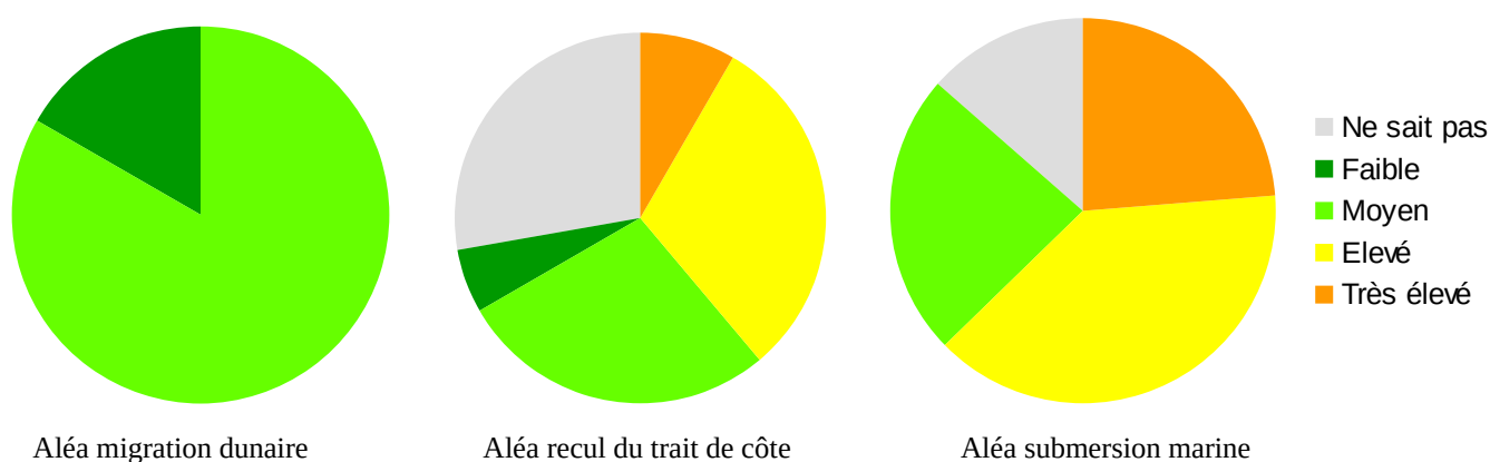
Figure 15. Niveaux de complexité de l'étude d'aléa migration dunaire, de l'aléa recul du trait de côte et de l'aléa submersion marine, estimés par les services de l'État
