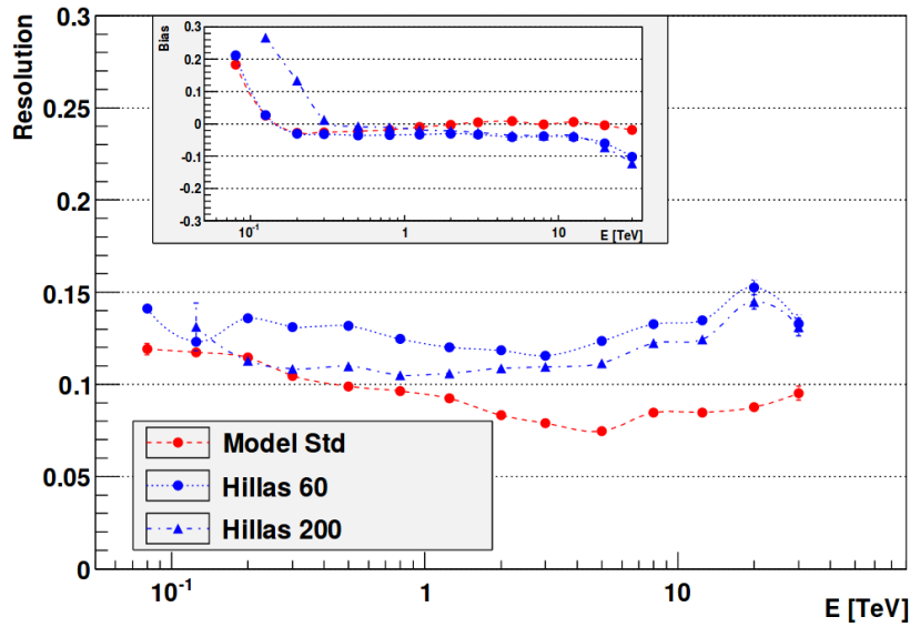
FIGURE 4.8 – Résolution en énergie en fonction de l'énergie pour des simulations de \gamma . Les cercles et triangles bleus représentent la résolution obtenue pour la méthode de Hillas pour deux jeux de coupures différents (respectivement « Hillas 60 » et « Hillas 200 »). Les cercles rouges représentent la résolution pour le modèle semi-analytique (« Model Std »). L'encart en haut à gauche représente le biais en énergie en fonction de l'énergie pour ces trois mêmes configurations d'analyse. Figure issue de [136].
