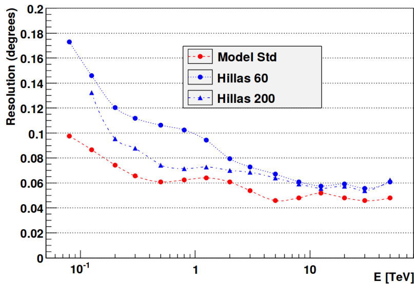
FIGURE 4.9 – Résolution angulaire en fonction de l'énergie pour des simulations de \gamma . Les cercles et triangles bleus représentent la résolution obtenue pour la méthode de Hillas pour deux jeux de coupures différents (respectivement « Hillas 60 » et « Hillas 200 »). Les cercles rouges représentent la résolution pour le modèle semi-analytique (« Model Std »). Figure issue de [136].
