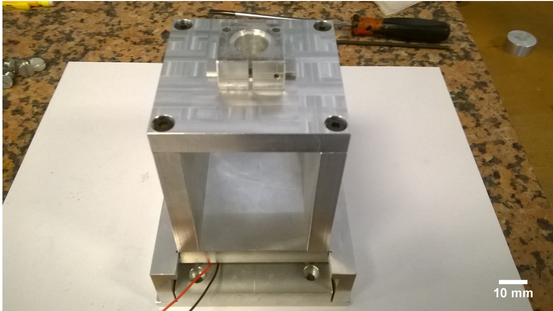
FIGURE 3.7 – Les trois pièces inférieures montées : fusible, arche et piston.
