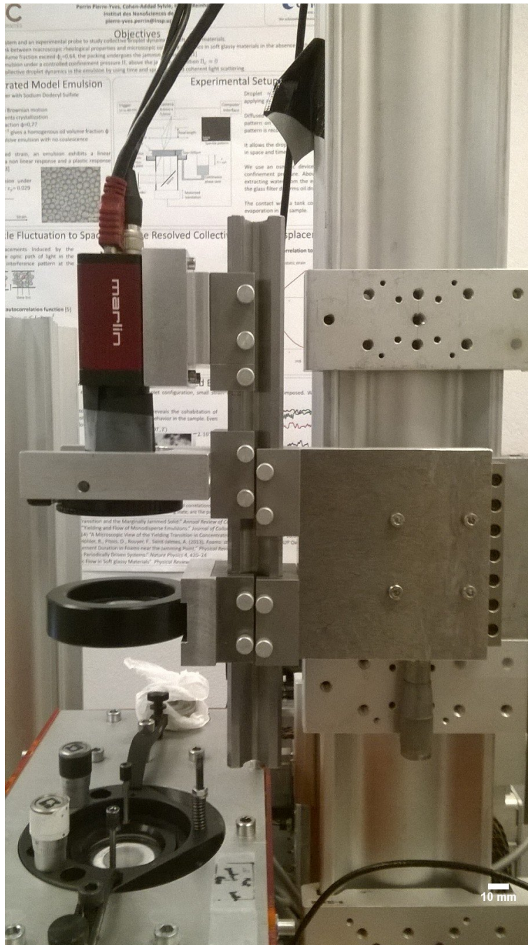
FIGURE 3.20 – Bloc de mesure optique.
