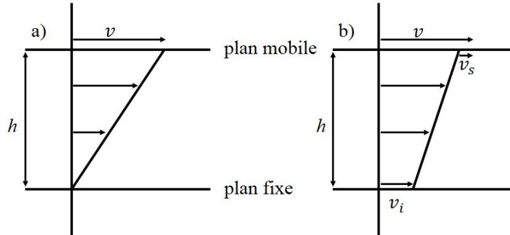
FIGURE 1.6 – Profil de vitesse dans un Couette plan : a) sans glissement aux parois, b) avec glissement aux parois
