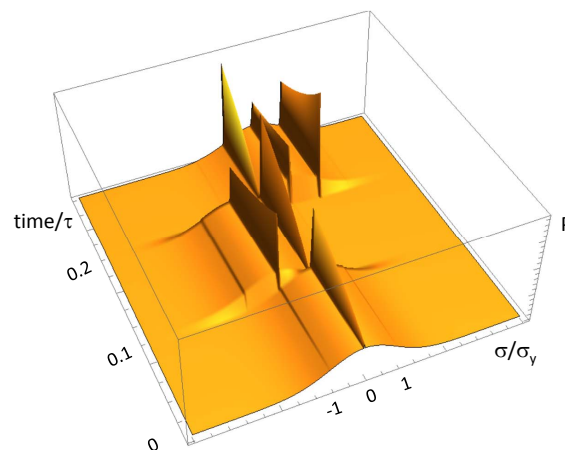
FIGURE 4.20 – Évolution temporelle de la distribution des contraintes de cisaillement, calculée pour le modèle de Hébraud et Lequeux, sous l’effet d’un cisaillement oscillatoire d’amplitude A_{PC} = \sigma_y/G (cf. figure 4.19). La condition initiale correspond à la gaussienne de largeur 2\sigma_y , illustrée sur la figure 4.18. Le paramètre de couplage \alpha_{HL} vaut 1.
