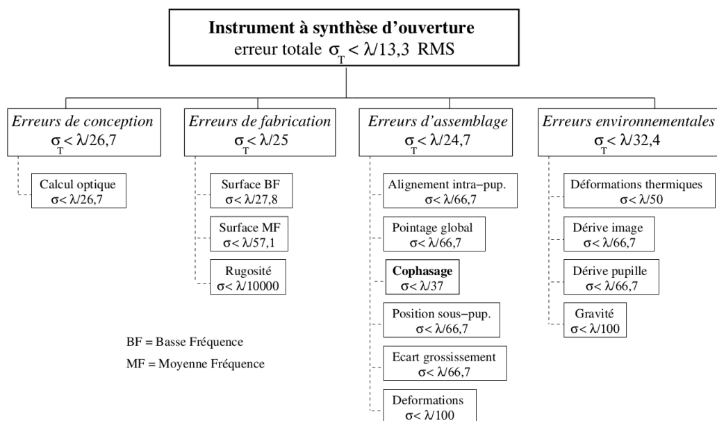
FIGURE 1.12 – Budget de qualité d’un instrument multi-pupille.
