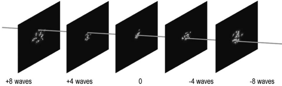
FIGURE 1.20 – Principe du GPR. Le rayon principal d’un segment, ou rayon passant par le centre du segment, va théoriquement passer par des pixels bien définis dans le cas aligné. Si le segment est désaligné, il s’agit de mesurer la distance entre le point d’impact théorique et le point d’impact effectif du rayon principal de chaque segment.
