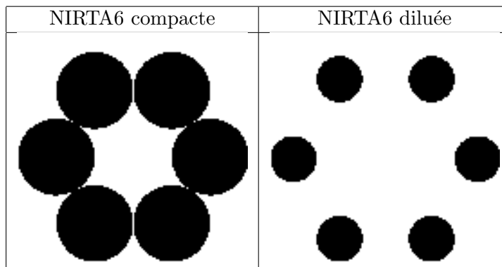
FIGURE 2.1 – Simulation d’une pupille à 6 sous-pupilles compacte (gauche) et diluée (droite).
