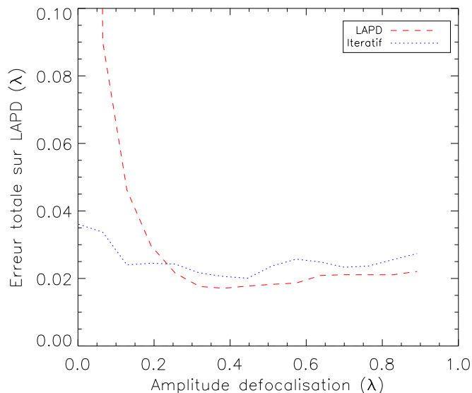
FIGURE 5.5 – Optimisation de la diversité de phase.
