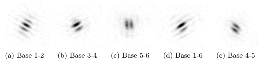
FIGURE 6.2 – Figures d'interférences entre différents segment du miroir NIRTA.
