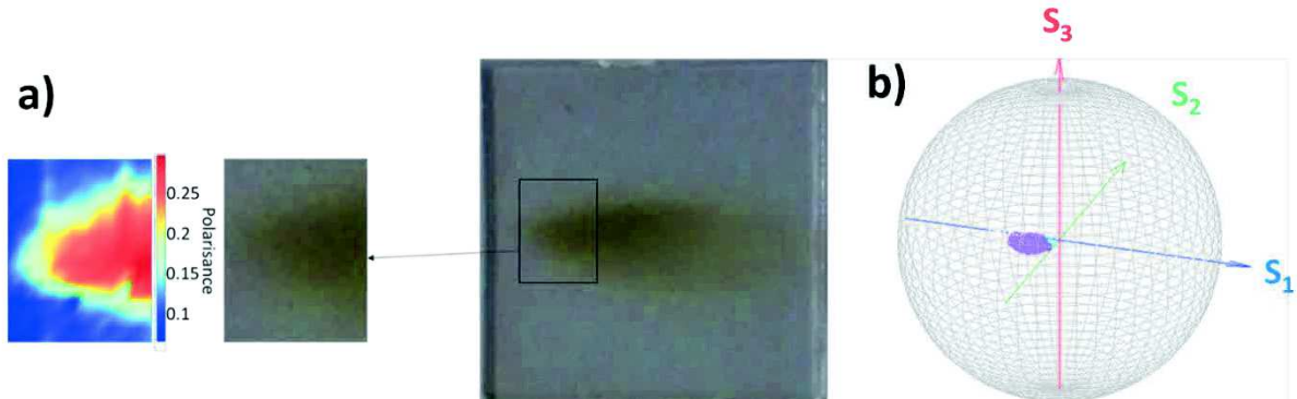
Figure 91 : (a) Cartographie de la polarisation à 645 nm sur une monocouche orientée de nanofils d'argent et photographie de la zone (b) Représentation dans la sphère de Poincaré des états de polarisations de la lumière transmise sous l'irradiation de lumière non polarisée par l'échantillon dans la zone étudiée. Les points représentés en magenta représentent la zone de dépôt tandis que les points en cyan représentent la zone extérieure au dépôt.
