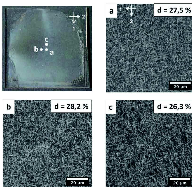
Figure 133 : Photographie d'un échantillon avec les des zones d'acquisition de clichés de microscopie électronique à balayage pour un film de deux couches orientées de nanofils d'argent dans des directions perpendiculaires.
