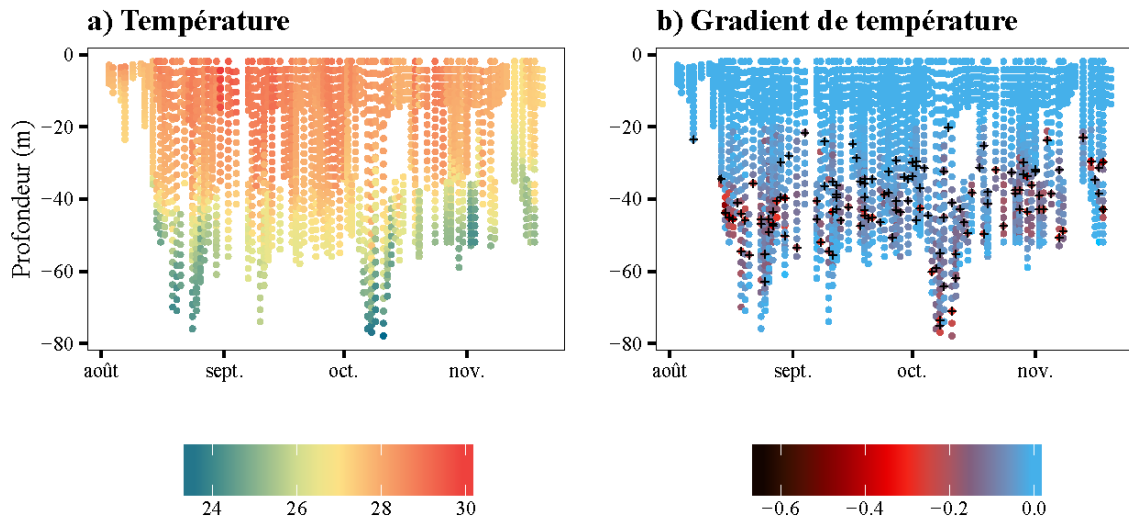
FIGURE 5.7 – (a) Profil de température ( ^{\circ}\text{C} ) de l'individu 135454 au cours du temps et (b) profil du gradient de température ( ^{\circ}\text{C}\cdot\text{m}^{-1} ) pour ce même individu. Les croix noires dans (b) correspondent aux profondeurs moyennes de chasse identifiées à l'aide du Hunting time .
