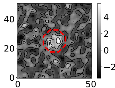
(b) Courbes de niveaux pour \sigma = 0.8
