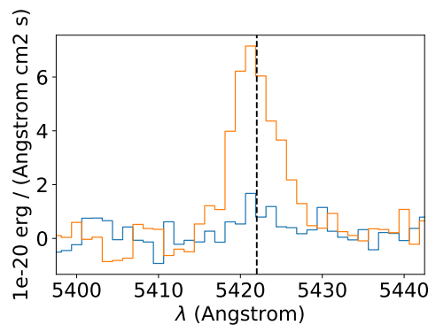
(e) Zoom autour de la raie. Spectres prétraités (soustraction continu et filtrage adapté spatial). En orange le spectre du pixel central de la galaxie, en bleu le pixel du halo
