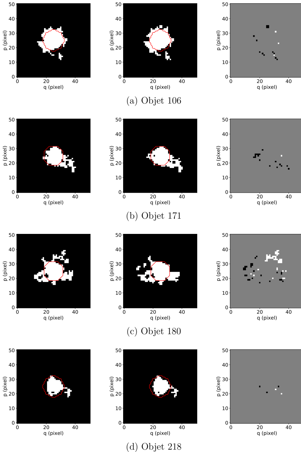
FIGURE 7.3 – Comparaisons des méthodes de soustraction de continu. À gauche : le résultat de détection en utilisant le filtre médian comme estimateur du continu ; au centre : le résultat de détection en utilisant la méthode de régression robuste développée en annexe B ; à droite : la différence entre les deux (les pixels noirs indiquent les détections obtenues uniquement en utilisant la méthode de régression robuste, les pixels blancs indiquent les détections obtenues uniquement en utilisant le filtre médian).
