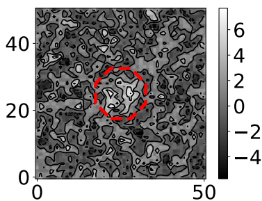
(a) Courbes de niveaux pour \sigma = 0.2
