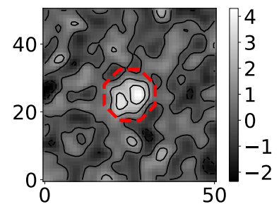
(c) Courbes de niveaux pour \sigma = 1.4
