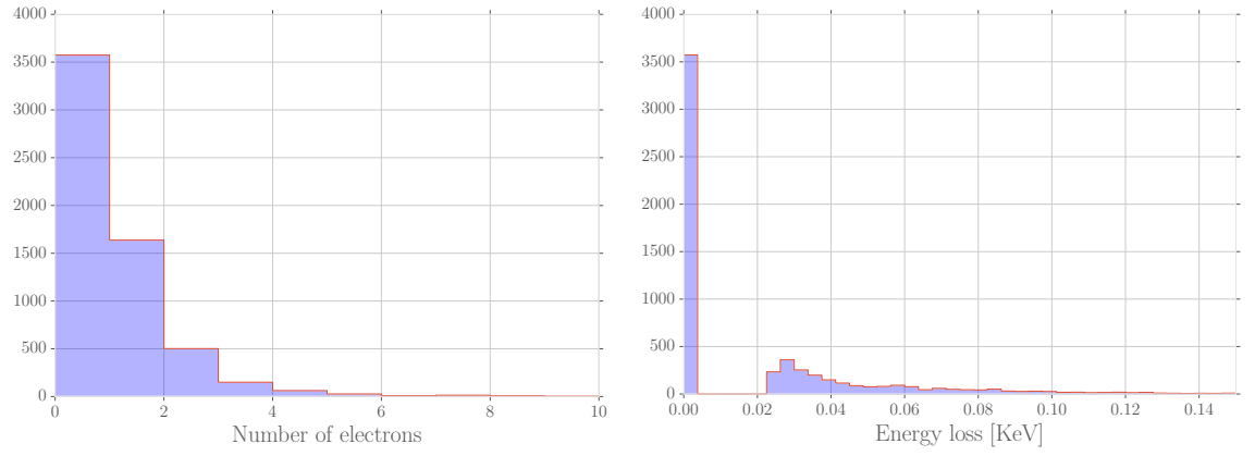
(b) Helium
