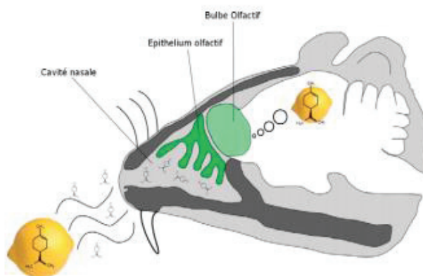
Figure 1. Système olfactif.
