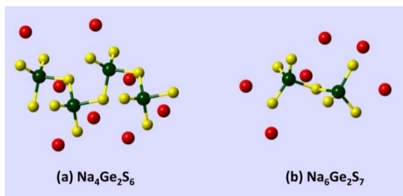
Figure IV.15. Structure cristallin de (a) Na 2 GeS 3 = Na 4 Ge 2 S 6 monoclinique, le groupe spatial P2 1 /c [48], et (b) Na 6 Ge 2 S 7 monoclinique, le groupe spatial C2/c [61]
