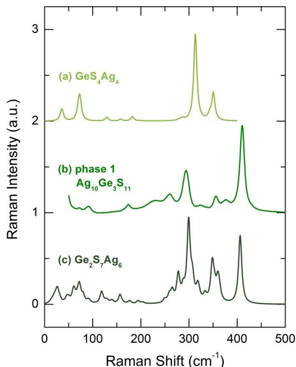
Figure IV.32. (a) Calcul DFT du spectre Raman de ISO- \text{GeS}_4\text{Ag}_4 , (b) spectre Raman expérimental de \text{Ag}_2\text{GeS}_3 recuit (phase 1 = \text{Ag}_{10}\text{Ge}_3\text{S}_{11} ) et (c) calcul DFT du spectre Raman des clusters CS- \text{Ge}_2\text{S}_7\text{Ag}_6 .
