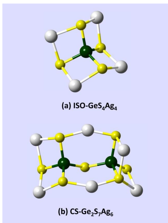
Figure IV.31. Structures optimisées de (a) tétraèdre isolé ISO- \text{GeS}_4\text{Ag}_4 et (b) dimère CS- \text{Ge}_2\text{S}_7\text{Ag}_6 utilisé pour la modélisation DFT. Les deux clusters représentent des motifs structuraux dans \text{Ag}_{10}\text{Ge}_3\text{S}_{11} .
