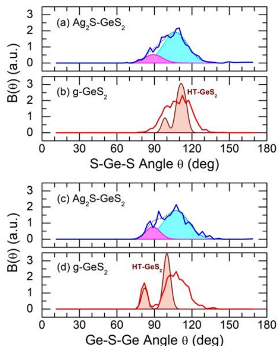
Figure IV.67. Distributions des angles de liaison dans (a,c) le verre (\text{Ag}_2\text{S})_{0.45}(\text{GeS}_2)_{0.55} et (b,d) \text{GeS}_2 cristallin et vitreux [84], [43]. Les dépendances angulaires S-Ge-S sont montrées dans les panneaux (a,b), Ge-S-Ge - dans les panneaux (c,d).
