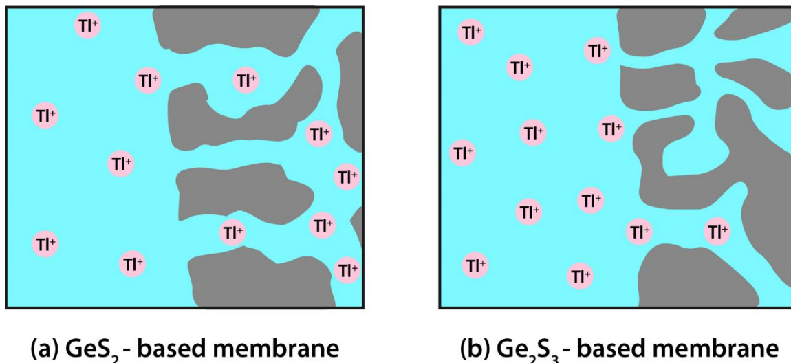
Figure V.33. Les membranes à base de \text{GeS}_2 (a) et \text{Ge}_2\text{S}_3 (b).
