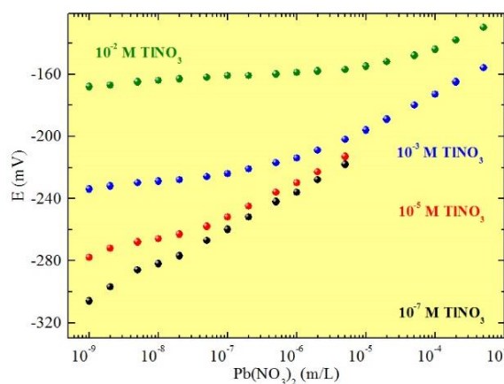
Figure V.22. Sélectivité de capteur 10Tl_2S-40Ag_2S-50GeS_2 en présence des ions interférents de Pb^{2+}
