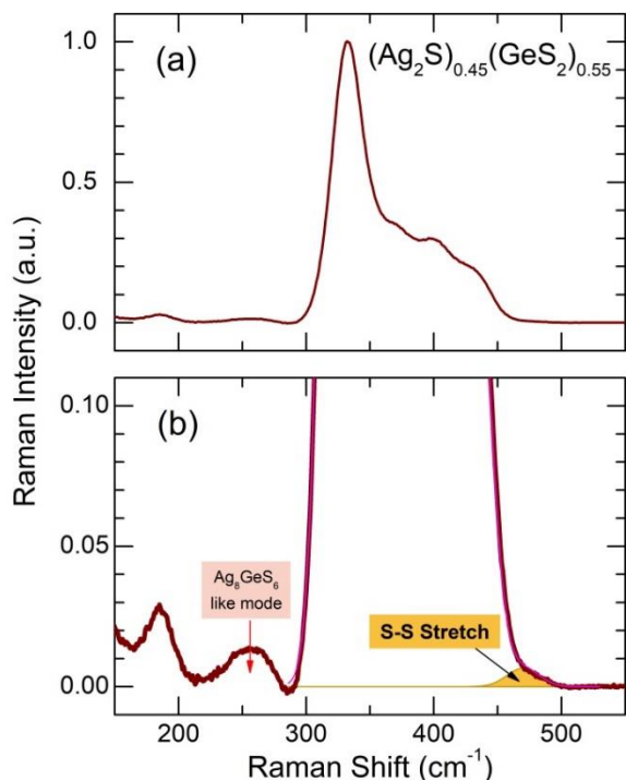
Figure IV.66. Spectre Raman expérimental du verre (\text{Ag}_2\text{S})_{0.45}(\text{GeS}_2)_{0.55} : (a) le spectre entier, (b) un détail montrant le mode d'élongation S-S (en jaune) et la caractéristique spectrale analogue à \text{Ag}_8\text{GeS}_8 .
