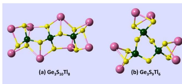
Figure IV.16. Structure optimisée des clusters oligomères connectés par sommet commun CS utilisés pour la modélisation DFT : (a) le trimère CS-Ge 3 S 10 Tl 8 et (b) l'anneau CS-Ge 3 S 9 Tl 6 .
