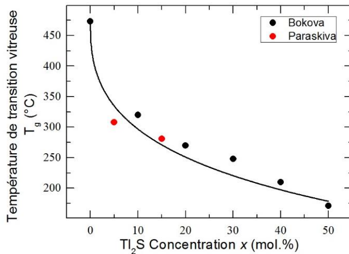
Figure I.17. Evolution de la température de transition vitreuse T_g dans le système (\text{Tl}_2\text{S})_x(\text{GeS}_2)_{100-x} en fonction du pourcentage molaire de \text{Tl}_2\text{S} . (•) Données obtenues lors de ce travail et (◦) données obtenues lors d'études réalisées précédemment au laboratoire.
