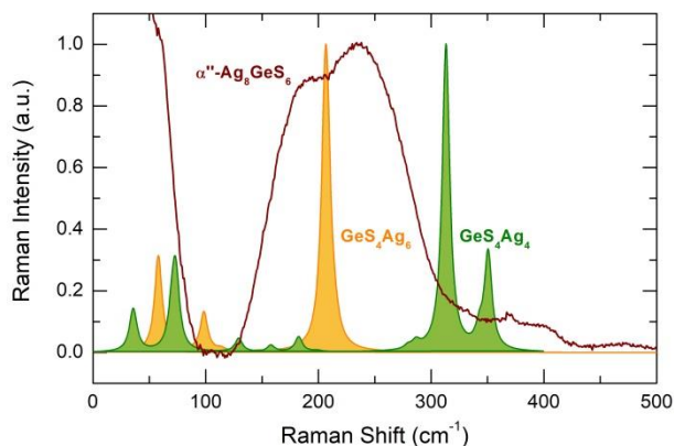
Figure IV.25. Spectres Raman DFT des clusters \text{GeS}_4\text{Ag}_4 (vert) et \text{GeS}_4\text{Ag}_6 (orange) par rapport aux données expérimentales pour \alpha'' - \text{Ag}_8\text{GeS}_6 orthorhombique.
