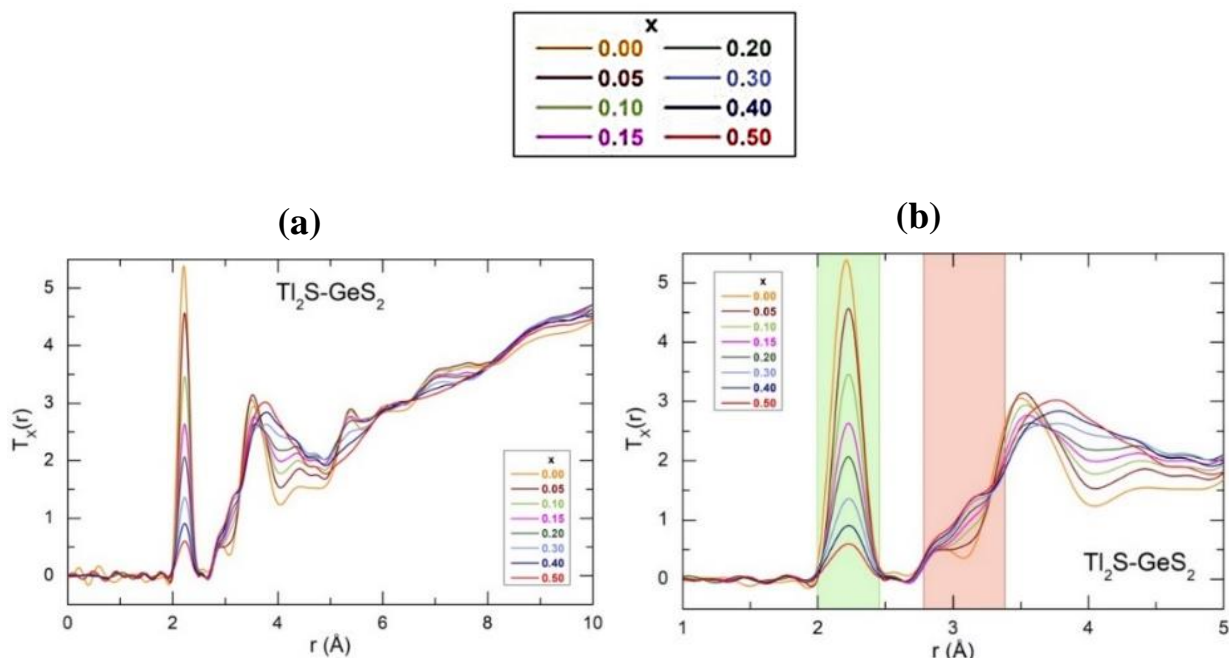
Figure IV.52. Les fonctions de corrélation totales obtenues avec les rayons X à haute énergie T_X(r) pour les verres (\text{Tl}_2\text{S})_x(\text{GeS}_2)_{1-x} : (a) l'espace r jusqu'à 10 Å, (b) la région de première et deuxième voisines; les corrélations de premier voisin Ge-S et Tl-S sont surlignées en vert et en rouge, respectivement.
