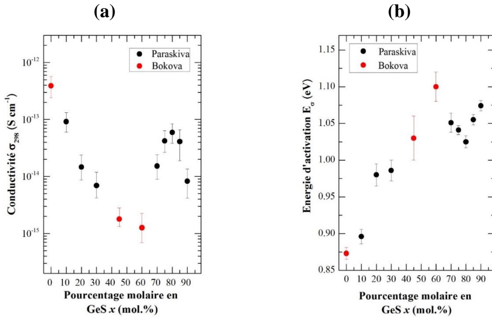
Figure II.25. (a) Conductivité à température ambiante \sigma_{298} , (b) l'énergie d'activation E_{\sigma} pour le système (\text{Tl}_2\text{S})_{10}(\text{GeS})_x(\text{GeS}_2)_{90-x} en fonction du pourcentage molaire de GeS. (•) Données obtenues lors de ce travail et (•) données obtenues lors d'études réalisées précédemment au laboratoire.
