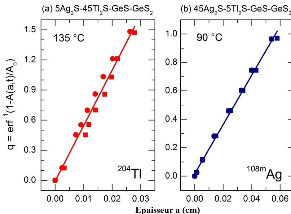
Figure III.3. Profils typiques des traceurs de diffusion (a) ^{204}\text{Tl} et (b) ^{108\text{m}}\text{Ag} des verres (\text{Ag}_2\text{S})_5(\text{Ti}_2\text{S})_{45}(\text{GeS})_{25}(\text{GeS}_2)_{25} et (\text{Ag}_2\text{S})_{45}(\text{Ti}_2\text{S})_5(\text{GeS})_{25}(\text{GeS}_2)_{25} recuits à 135^\circ\text{C} et à 90^\circ\text{C} , respectivement.
