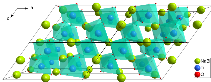
Figure 29 : Représentation de la maille monoclinique de NBT [133]
