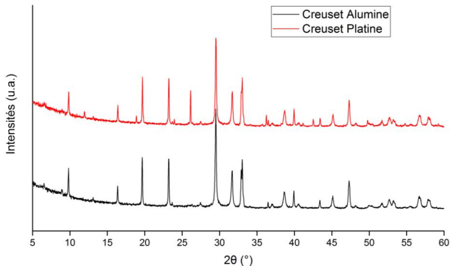
Figure 48 : Comparaison des résultats des calcinations réalisées en creuset alumine et platine
