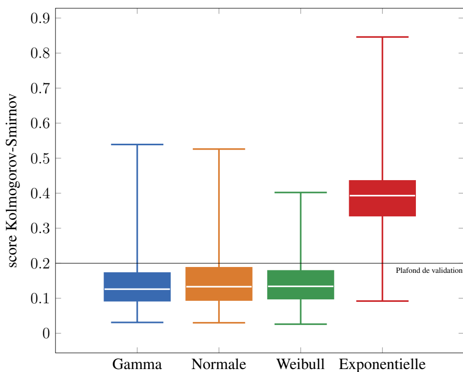
FIGURE 6.3 – Répartition des scores pour chaque loi
