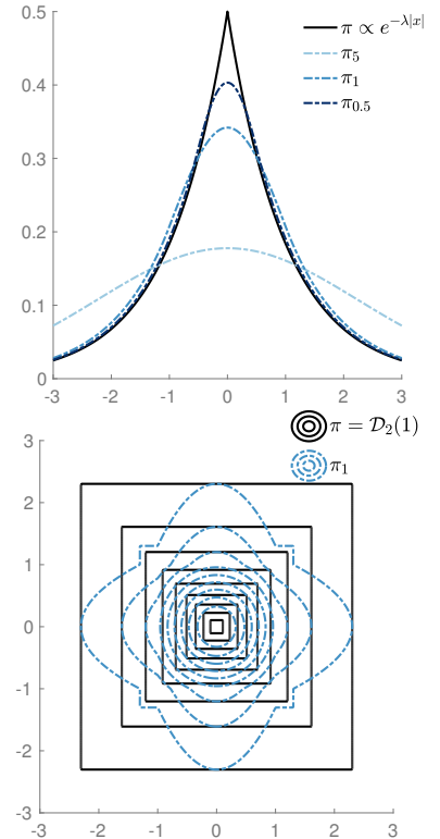
FIGURE 2.7 : Haut : approximations de moreau de \pi = \mathcal{D}_1(1) pour plusieurs valeurs de \delta . Bas : Lignes de niveau de \pi = \mathcal{D}_2(1) (noir) et de son approximation de Moreau pour \delta = 1 .
