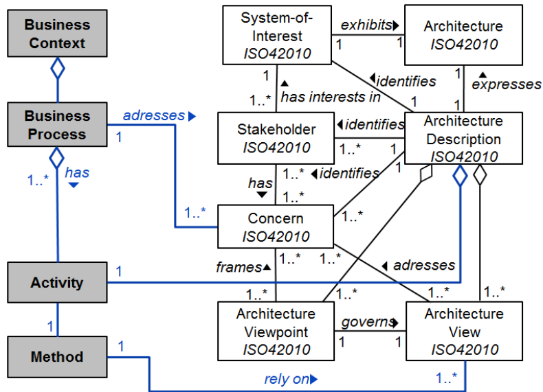
Figure 14 Relation entre le contexte d'une discipline d'ingénierie et les modèles d'architecture
