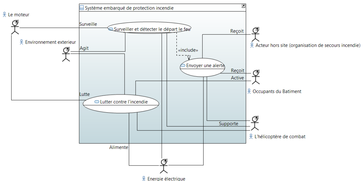
Figure 88 Diagramme UML de cas d'utilisation du système
