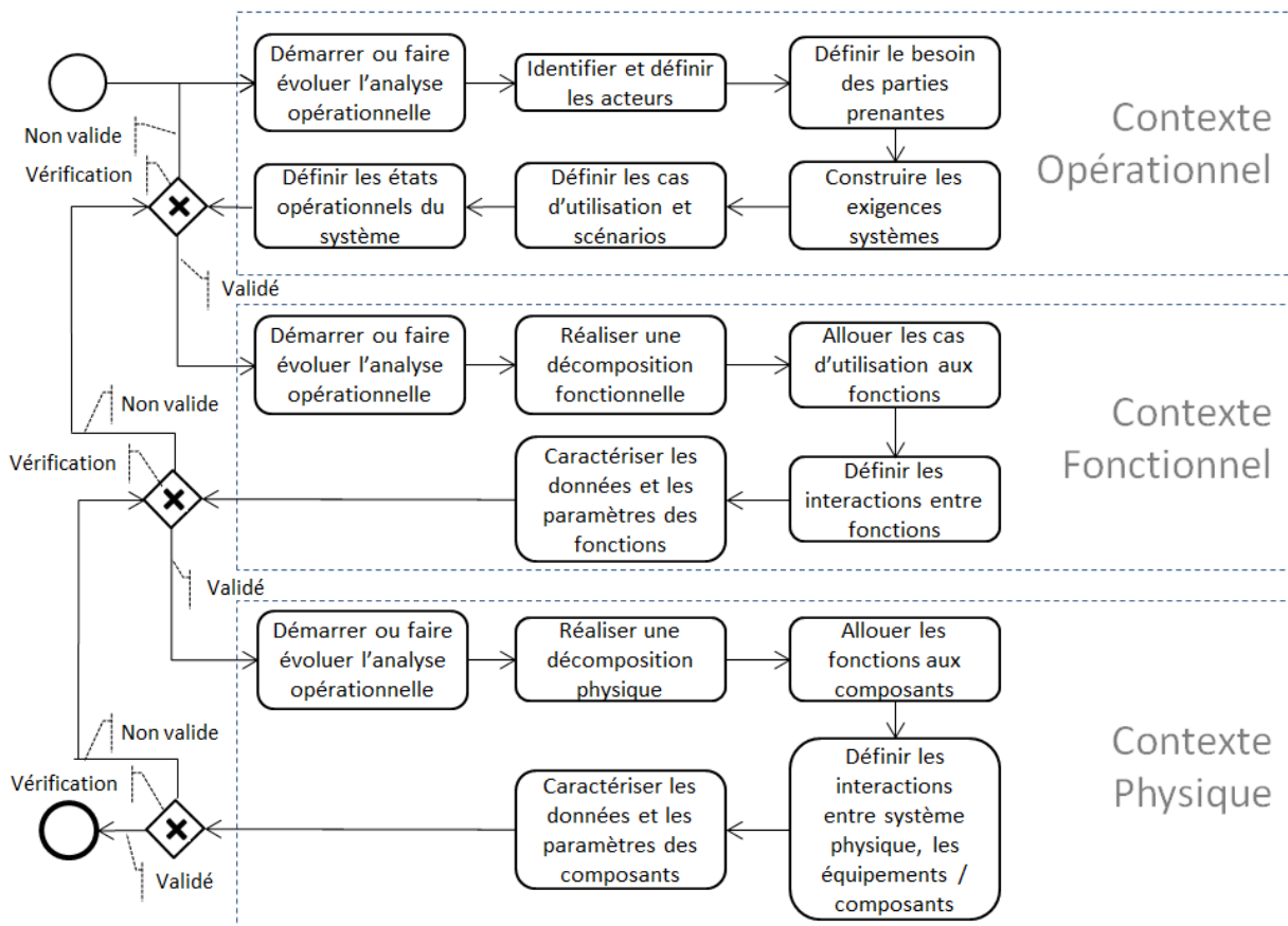
Figure 86 Diagramme BPMN du processus de l'Équipementier A de l'architecture système
