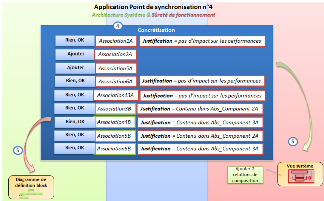
Figure 178 Application de la concrétisation du point de synchronisation n°4
