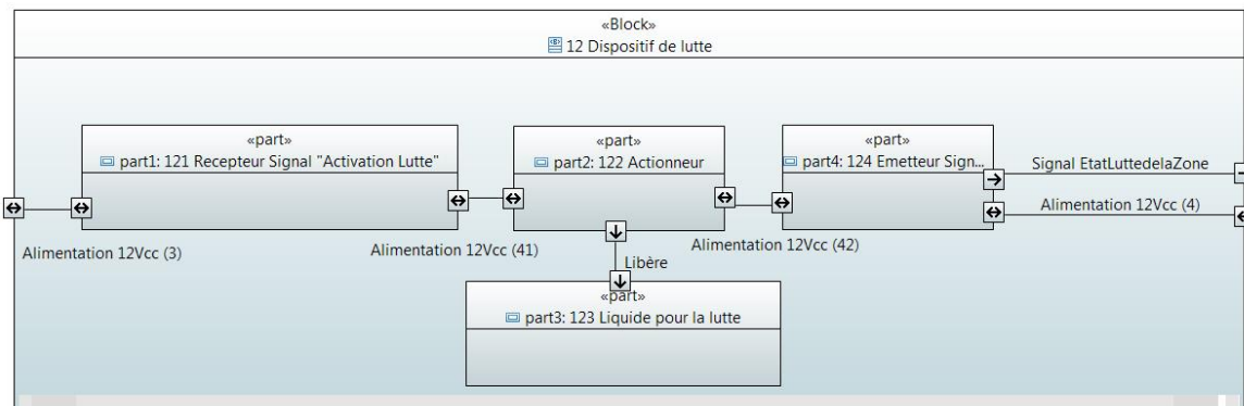
Figure 100 Interaction des composants du sous-système dispositif de lutte
