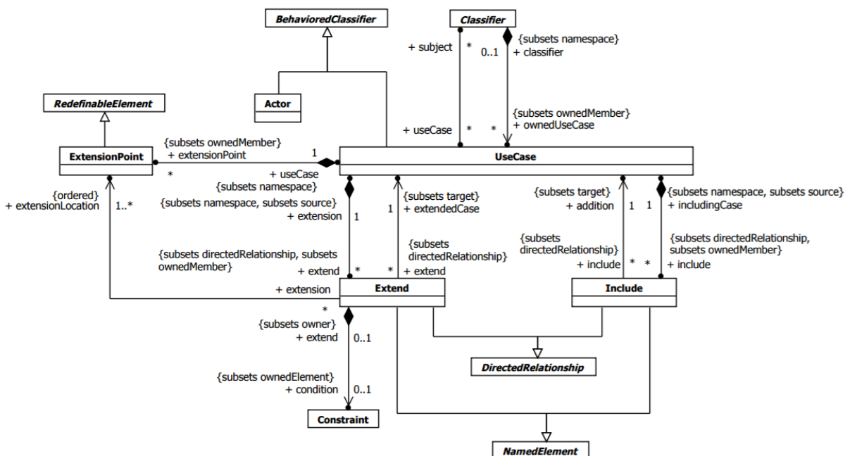
Figure 58 Métamodèle UML du diagramme cas d'utilisation
