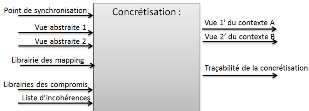
Figure 39 Fonction de concrétisation de la synchronisation
