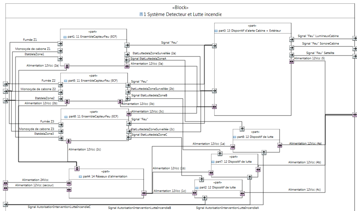
Figure 96 Interactions des sous-systèmes dans un diagramme de blocks internes
