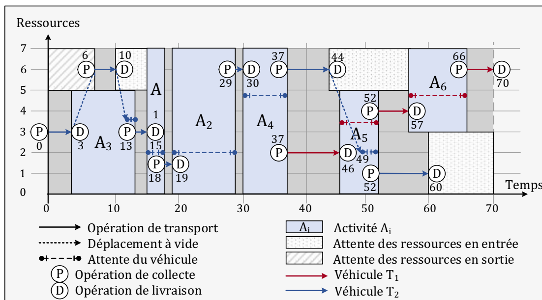
Figure 4-35. Solution optimale de l'instance LMQV_C1 du RCPSPR
