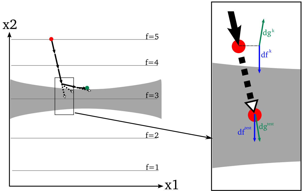
Figure A.1 – Exemple de problème d'optimisation à deux paramètres (x_1, x_2) sous une contrainte représentée par la zone grise. L'algorithme MFD classique, si le pas est trop faible, va rester bloquer au point vert. L'agrandissement de droite va servir de base pour la notion de permissivité.
