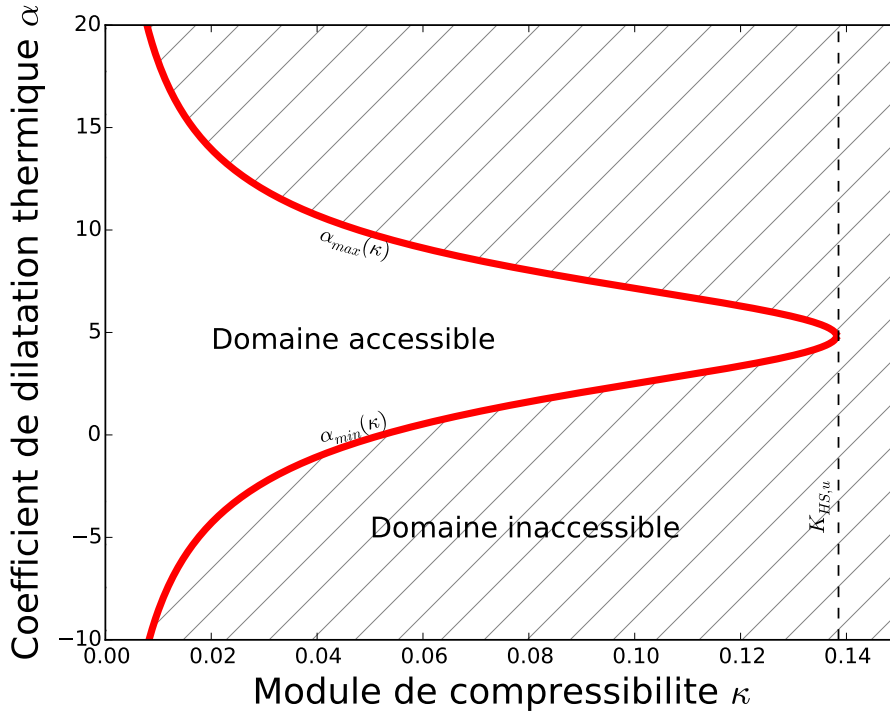
Figure B.1 – Forme typique des bornes de Gibiansky-Torquato pour un matériau quelconque, la courbe formée délimite deux espaces de propriétés accessible et inaccessible par un matériau isotrope. La borne supérieure de Hashin-Strikeman pour le module de compressibilité a aussi été ajoutée sur la figure.
