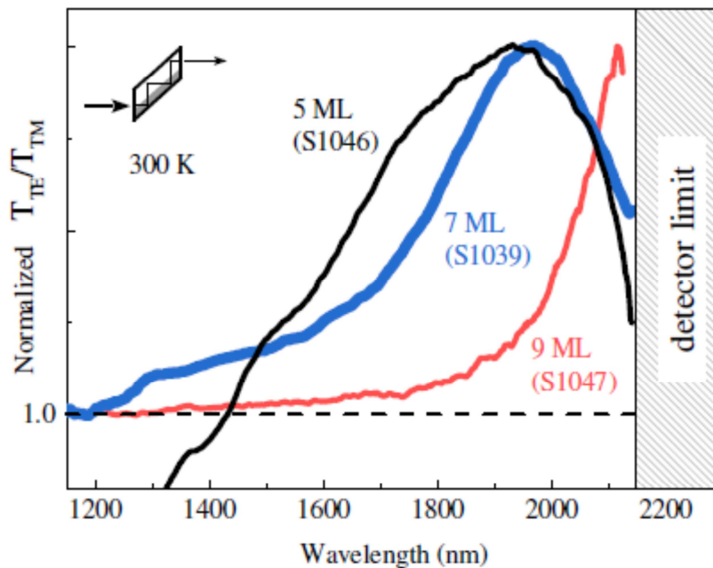
Fig 3.20 : Effet de l'épaisseur des puits sur le spectre l'anisotropie d'absorption normalisée[56].
