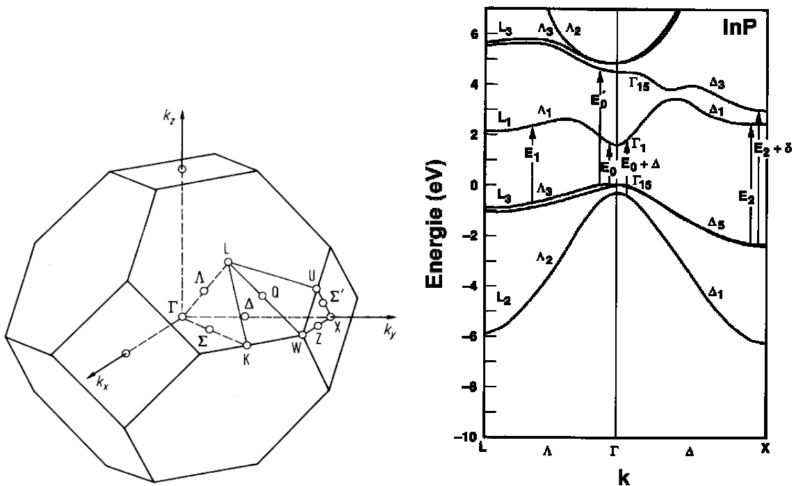
Fig.1.27 : Zone de Brillouin pour une structure de type zinc-blende et exemple de diagramme de bandes associé (ici InP)
