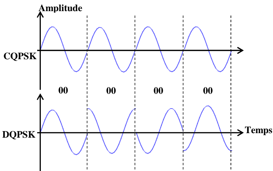
Fig1.12 : Comparaison de deux segments de signaux QPSK et DQPSK
