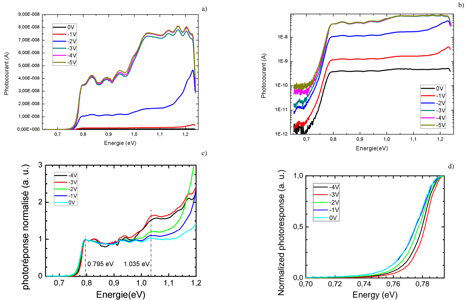
Fig.3.26 : Mesure de photocourant sur S1353 p6 à 300K. Données brutes en échelle linéaire (a) et semi-logarithmique (b) ainsi que mesure normalisée à 0.795eV (c) avec vue rapprochée sur l'élargissement du front d'absorption en fonction de la tension (d).
