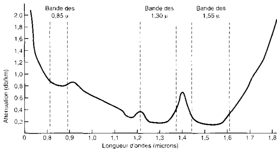
Fig1.3 : Le tracé de l'atténuation (absorption) dans la silice met en évidence trois bandes adaptées à la transmission optique dans l'infrarouge, en particulier les fenêtres centrées à 1.3 et 1.55 \mu m seront exploitées dans la transmission par fibre optique. Le pic situé à 1.4 \mu m correspond à l'absorption des liaisons OH, et est lié la technologie d'élaboration employée [18].
