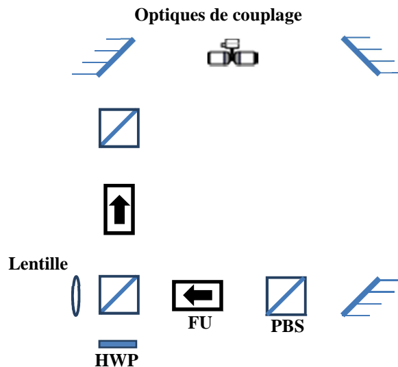
Fig.2.16 : Schémas de la boucle Sagnac mise en place.
