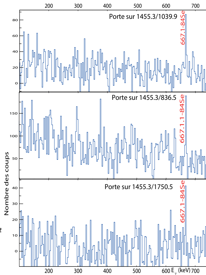
(b) Spectres en énergie pour les raies \gamma en coïncidence entre 100 et 750 keV.
