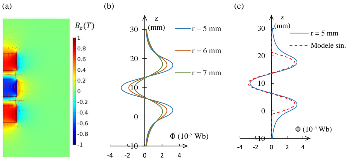
FIGURE 3-11 – Exemple de chaîne de 3 aimants alternés (aimant unité de dimensions \varnothing 8 mm x h 5mm et magnétisation N45). Les disques intercalaires ferromagnétiques ( \varnothing 7 mm x h 2.5mm) ont une perméabilité magnétique relative \mu_r=1000 . (a) Simulation FEM COMSOL – Composante axiale B_z du champ magnétique. (b) Flux magnétique capturé par une spire circulaire coaxiale avec la chaîne d'aimants, en fonction de sa position z et de son rayon r . (c) Modèle sinusoïdal du flux magnétique utilisé pour les optimisations des démonstrateurs.
