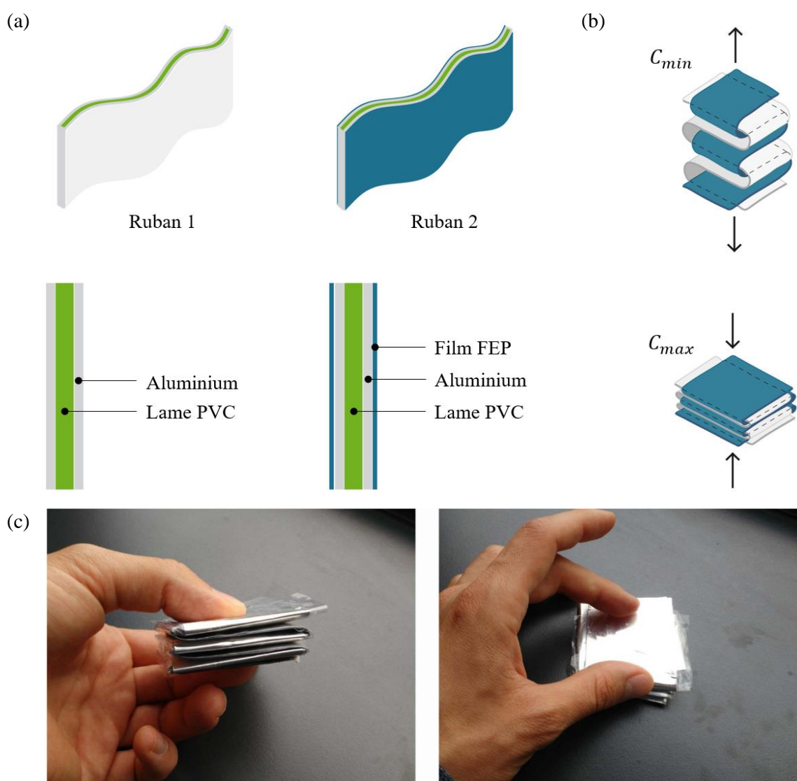
FIGURE 5-11 – Prototype de capacité variable triboélectrique. (a) Structure des deux électrodes. (b) Assemblage et configurations capacitatives extrémales. (c) Photographies du dispositif.
