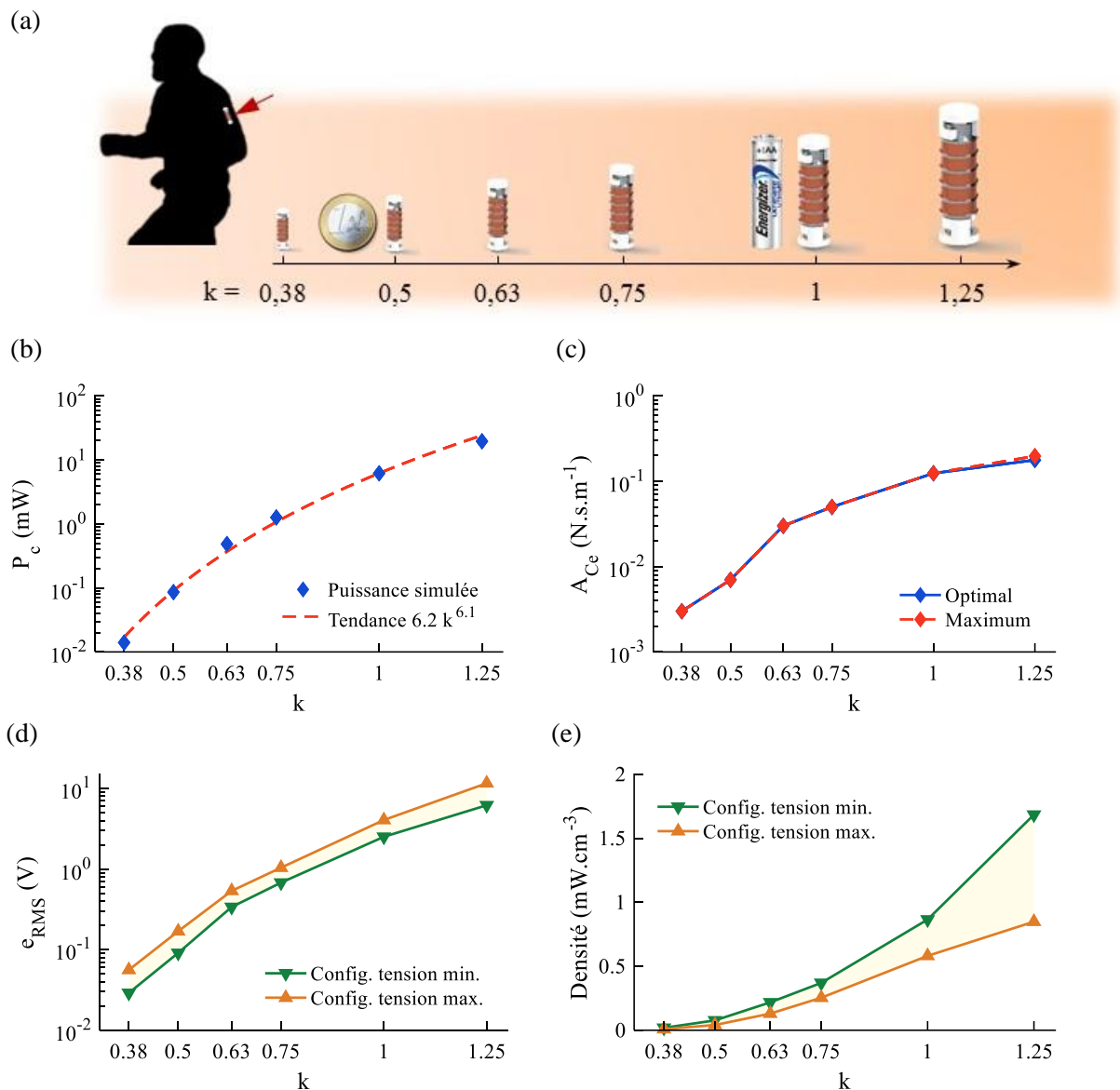
FIGURE 3-25 – Simulation (entrée de type « course à 4.8 km/h ») – Etude d'échelle. (a) Facteurs d'échelle k considérés. (b) Puissance électrique optimale dans la charge résistive ( 2 \times R_c ) (c) Amplitude de l'amortissement électrique A_{Ce} (maximum and optimum). (d) Force électromotrice e (RMS) des bobines et (e) densité de puissance, pour les configurations de bobinages possibles correspondant aux extrema de tension et associés à la puissance optimale.
