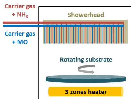
Fig. 2.9 – growth chamber of AIXTRON CRIUS.
