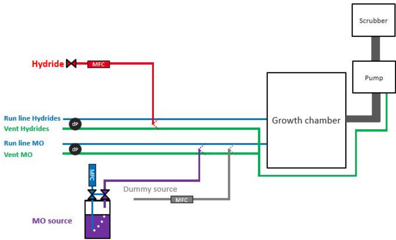
Fig. 2.8 – Gas lines in AIXTRON Crius.
