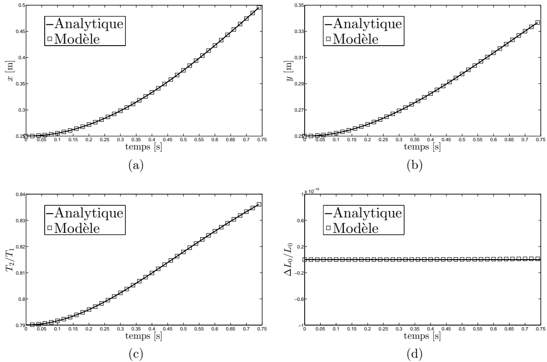
FIGURE 4.8 – Comparaison entre les solutions analytiques et les solutions obtenues par simulation numérique à l'aide du modèle de câble glissant pour le mécanisme de glissement théorique : (a) position horizontale; (b) position verticale; (c) ratio des tensions; (d) variation relative de la longueur neutre totale
