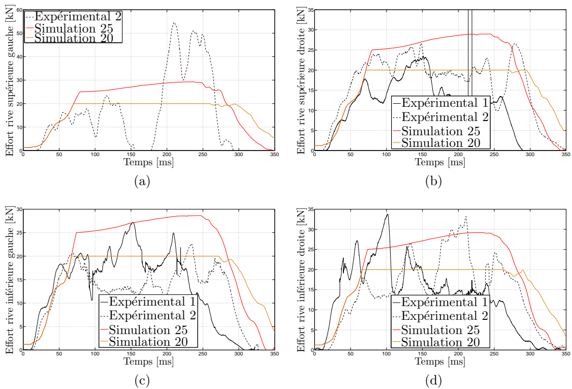
FIGURE 5.23 – Efforts dans les câbles de rive de l’ouvrage C2ROP lors de l’essai d’impact unique, influence du comportement des dissipateurs d’énergie : (a) câble de rive supérieure gauche ; (b) câble de rive supérieure droite ; (c) câble de rive inférieure gauche ; (d) câble de rive inférieure droite
