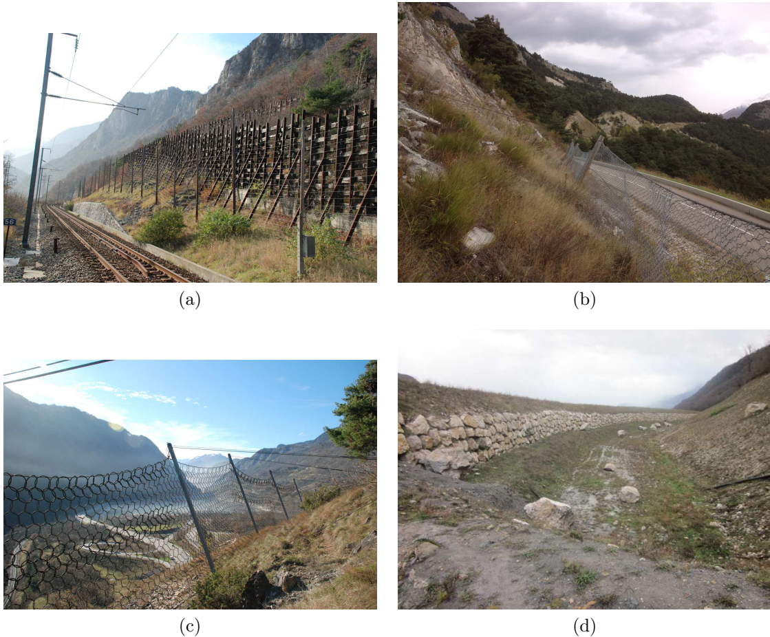
FIGURE 1.4 – Parades passives : (a) barrière rigide de rails et de traverses en bordure de voie de chemin de fer ; (b) barrière grillagée en pied de versant ; (c) écrans de filets ; (d) merlon avec blocs dans la fosse (source Cerema)
