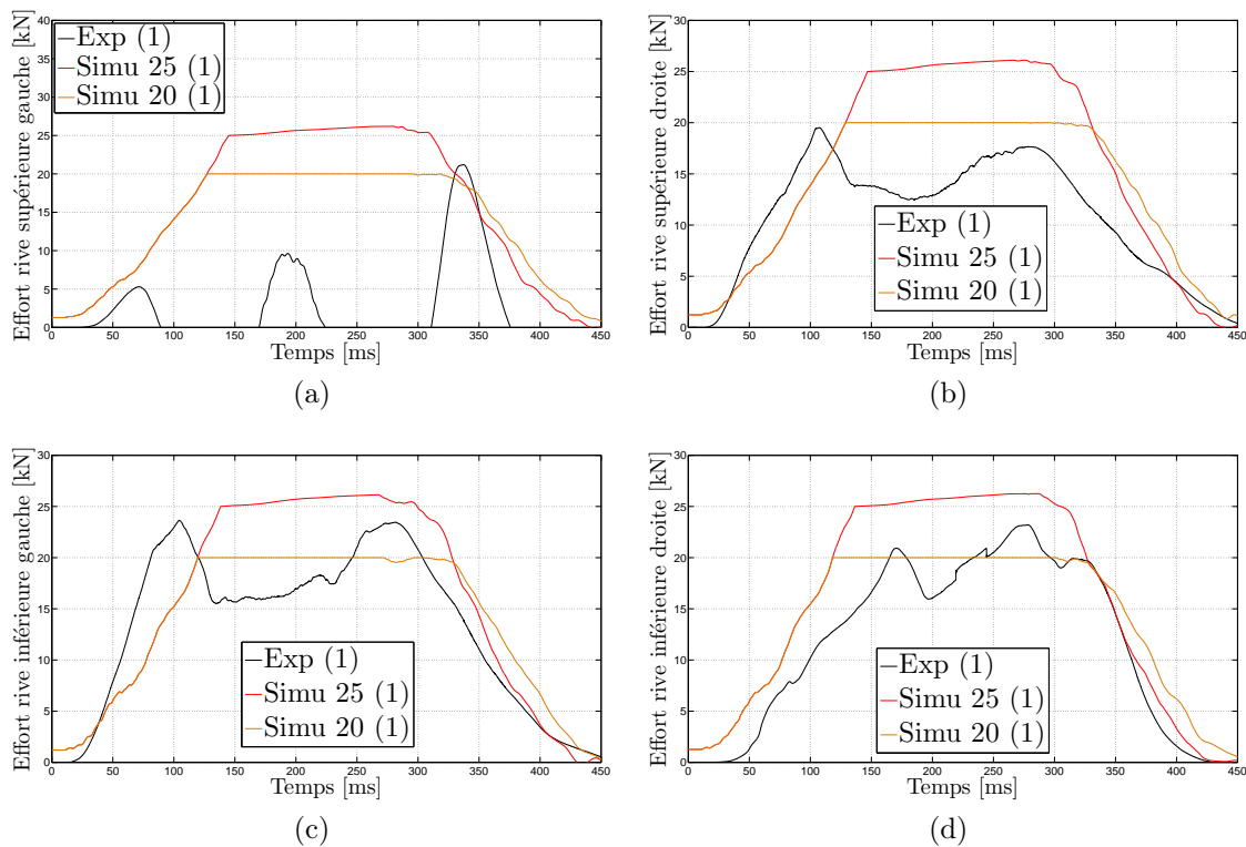
FIGURE 5.27 – Efforts dans les câbles de rive de l'ouvrage C2ROP lors du premier impact de l'essai d'impacts répétés : (a) câble de rive supérieure gauche ; (b) câble de rive supérieure droite ; (c) câble de rive inférieure gauche ; (d) câble de rive inférieure droite
