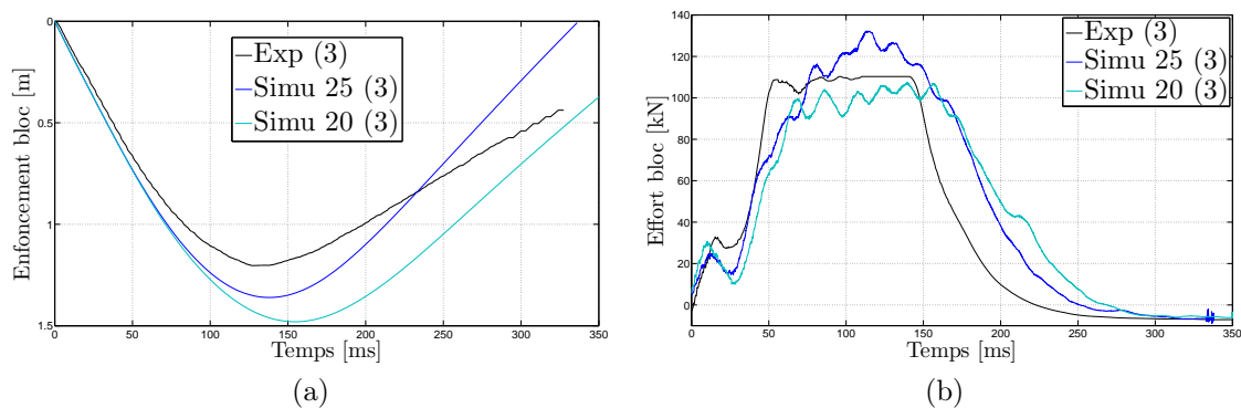
FIGURE 5.32 – Réponse globale de l'ouvrage C2ROP lors du troisième impact de l'essai d'impacts répétés : (a) enfoncement du bloc ; (b) effort total appliqué au bloc
