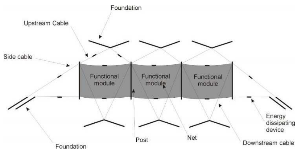
FIGURE 1.7 – Vue arrière d'un écran de filets contre les chutes de blocs rocheux (source [EOTA, 2013])
