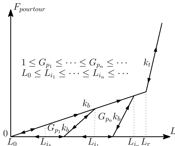
FIGURE 3.4 – Loi de comportement de la liaison de pourtour
