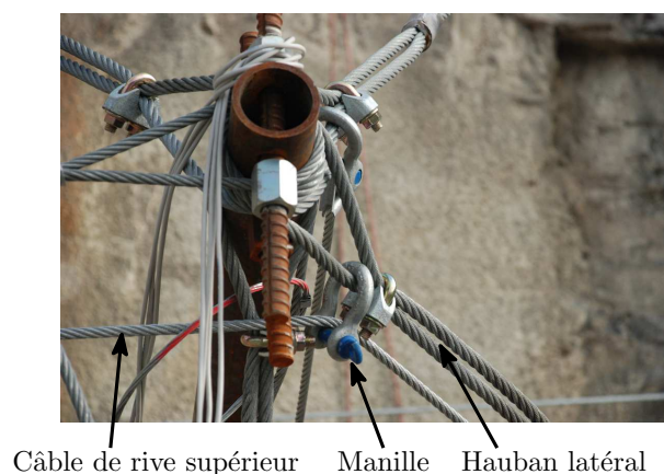
FIGURE 5.16 – Détail d'assemblage de la tête de poteau de l'écran C2ROP
