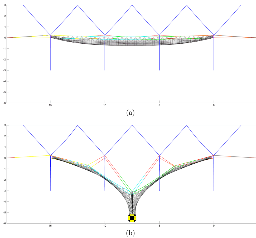
FIGURE 5.12 – Évolution temporelle de l'ouvrage C2ROP lors de la simulation numérique de l'essai quasi-statique : (a) état initial ; (b) allongement maximal ;
