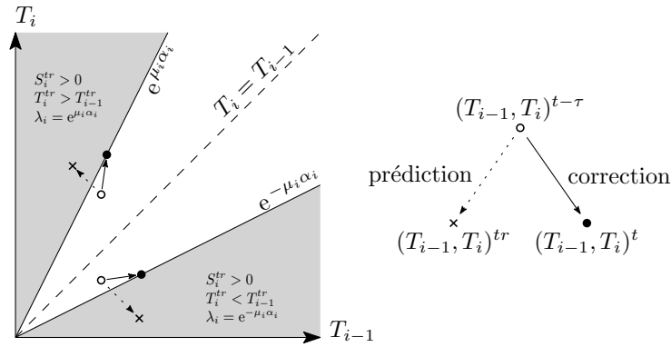
FIGURE 4.5 – Tensions dans les segments adjacents à un nœud glissant : tensions admissibles (blanc) et tensions dépassant la limite de glissement (gris)
