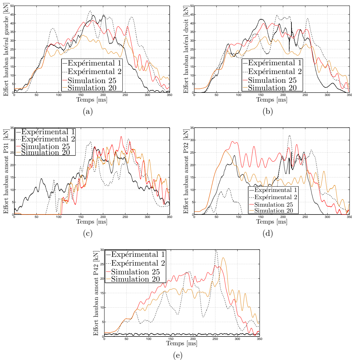
FIGURE 5.22 – Efforts dans les haubans de l'ouvrage C2ROP lors de l'essai d'impact unique, influence du comportement des dissipateurs d'énergie : (a) hauban latéral gauche ; (b) hauban latéral droit ; (c) hauban amont P31 ; (d) hauban amont P32 ; (e) hauban amont P42
