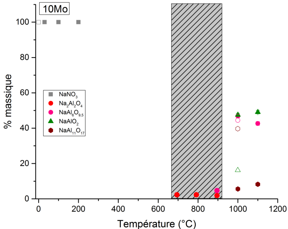
Figure 67 : Evolution des fractions cristallines déterminées par affinement Rietveld en fonction de la température du calcinat C-10Mo (normalisées sans tenir compte de la fraction amorphe). Les symboles évidés correspondent aux quantifications renormalisées sans amorphe, Al(OH)_3 , Na_2MoO_4 anhydre et hydraté, obtenues par DRX ex-situ à la température ambiante et à 1000 °C.
