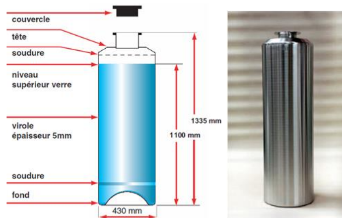
Figure 3 : Conteneur Standard de Déchets Vitriifiés CSD-V [27].
