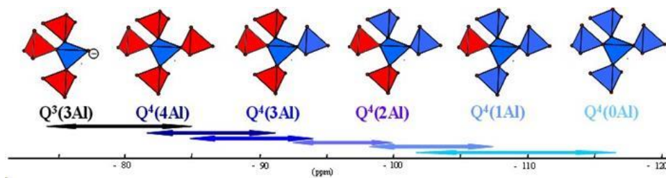
Figure 17 : Représentation des unités Q^4(mAl) et Q^3(mAl) : les tétraèdres de silicium sont en bleu par rapport aux tétraèdres d'aluminium en rouge.
