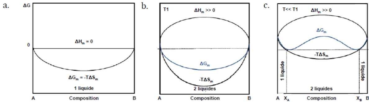
Figure 27 : Variations de l'enthalpie libre \Delta G_m du mélange binaire A-B dans le cas (a) d'une solution idéale, (b) et (c) d'une solution instable dépendante de la variation de l'entropie \Delta S_m du mélange. Dans le cas (b), l'entropie est maximale avec T_1 une température élevée et dans le cas (c), l'entropie est plus faible et T < T_1 [56].
