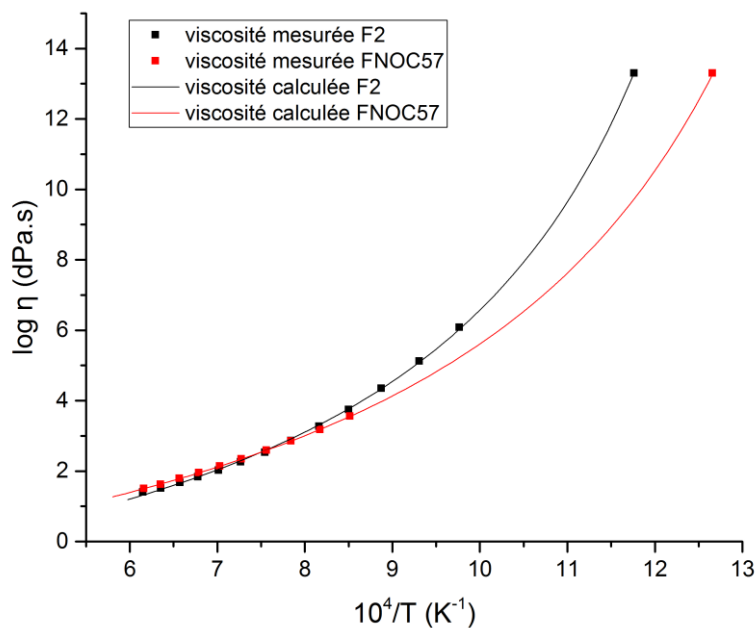
Figure 102 : Viscosité des frites de verre en fonction de la température. Ces courbes sont obtenues à l'aide d'une équation VFT.
