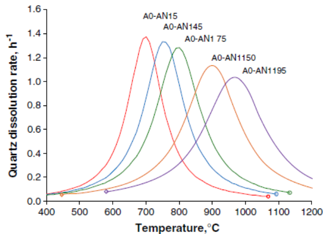
Figure 40 : Taux de dissolution du quartz dans les mélanges du groupe A0-ANI pour des tailles de particules initiales de 5, 45, 75, 150 et 195 µm (de gauche à droite) [108].
