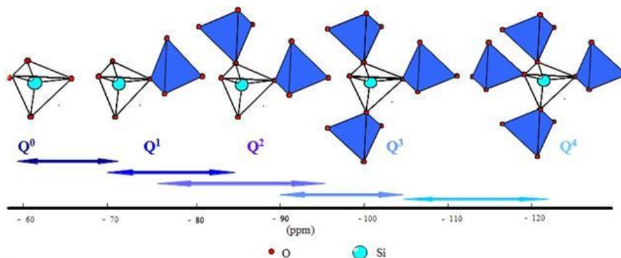
Figure 13 : Représentation des différentes configurations structurales Q^n ainsi que leur gamme de déplacements chimiques associée (en ppm).
