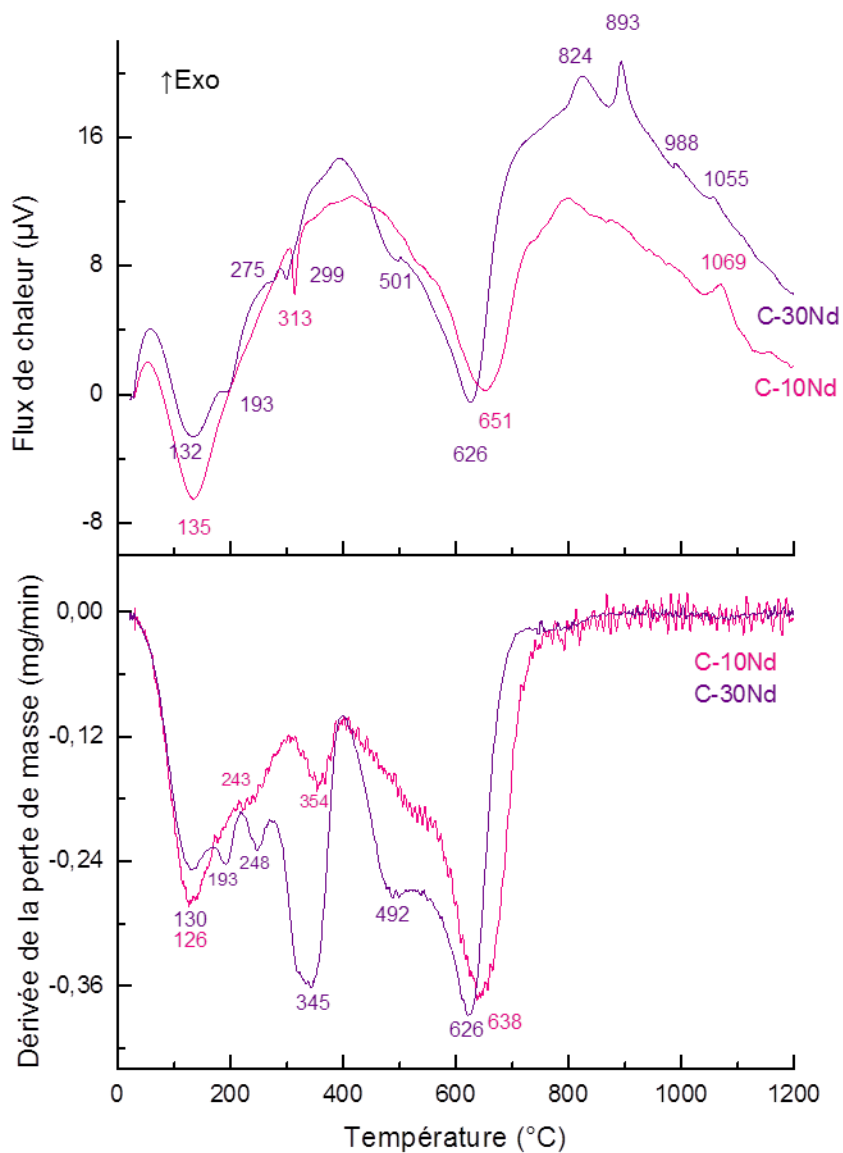
Figure 84 : Analyses thermiques différentielles et thermogravimétriques des calcinats C-10Nd et C-30Nd.
