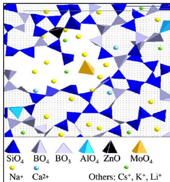
Figure 25 : Représentation structurale montrant l'incorporation du molybdène dans les zones dépolymérisées d'un verre de type aluminoborosilicate de sodium d'après des résultats de dynamique moléculaire et de spectroscopie EXAFS [47].
