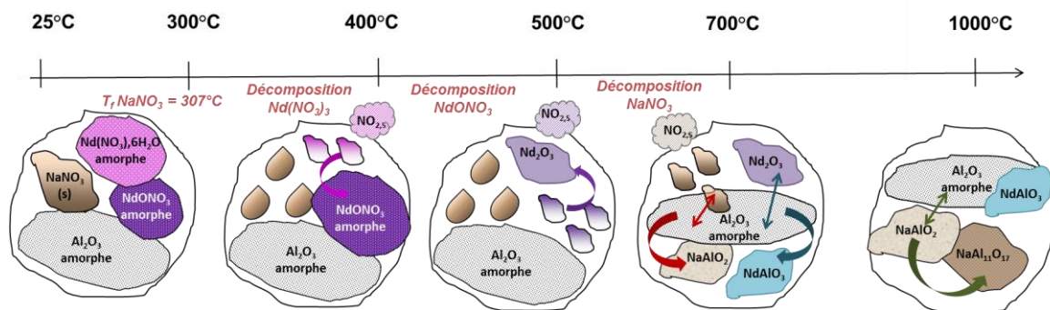
Figure 95 : Schématisation du mécanisme de transformation d'un calcinat appartenant au système (Na 2 O-Al 2 O 3 -Nd 2 O 3 ) lors d'une élévation de température de 25 °C à 1000 °C.
