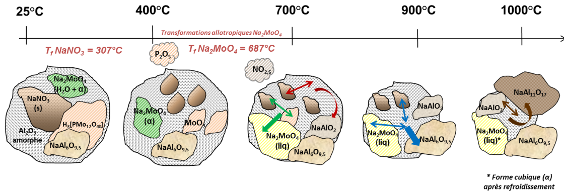
Figure 94 : Schématisation du mécanisme de transformation d'un calcinat appartenant au système (Na 2 O-Al 2 O 3 -MoO 3 ) lors d'une élévation de température de 25 °C à 1100 °C.
