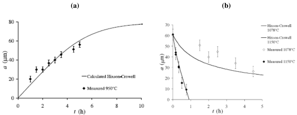
Figure 35 : Evolution de la taille du cristal de spinelle mesurée et calculée en fonction du temps (a) lors de la croissance du cristal à 950 °C et (b) lors de la dissolution à 1150 °C et 1078 °C [105].
