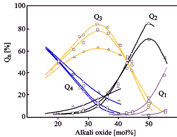
Figure 14 : Evolution de la distribution des entités Q^n au sein des verres SiO_2-M_2O en fonction de la teneur en oxyde alcalin M_2O ( \Delta=Li ; \square=Na ; \circ=K ) selon Maekawa et al. [8](avec F_k < F_{Na} < F_{Li} ).
