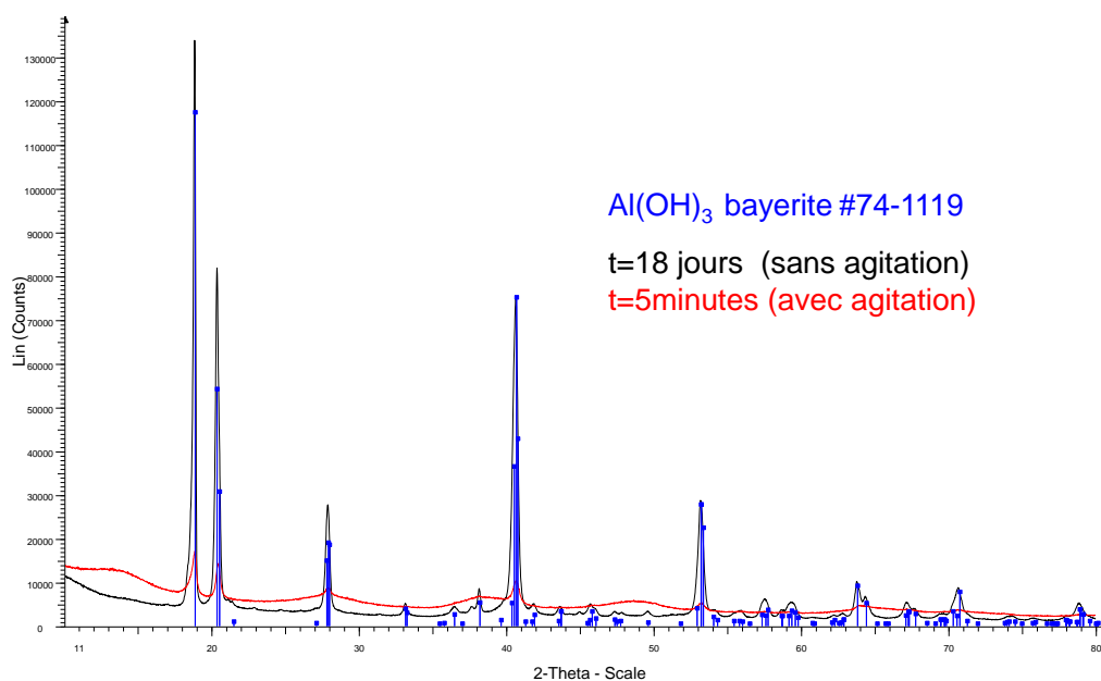
Figure 74 : Mise en évidence de l'hydratation de \text{NaAlO}_2 en \text{Al(OH)}_3 par Diffraction des Rayons X. Tests réalisés à température ambiante à partir d'un mélange de \text{NaAlO}_2 commercial et d'eau ultra pure avec ou sans agitation et en fonction du temps. Le précipité a été filtré puis séché à 120 °C pendant une nuit.
