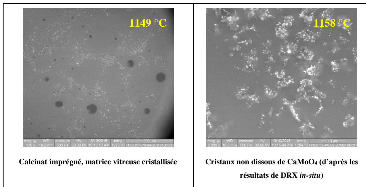
Figure 129 : Images acquises par microscopie électronique à balayage environnemental in-situ en température pour le mélange entre la fritte FNOC57 et le calcinat C-20Mo-10NdTT avec un rapport masse fritte/masse de verre (F/V) de 0,89 (rampe 50 °C/min ; sous air, avec une pression de 500 Pa).
