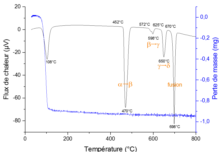
Figure 73 : Analyses thermiques différentielles et thermogravimétriques du composé Na 2 MoO 4 pur.
