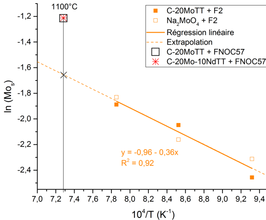
Figure 141 : Comparaison des conditions de saturation des phases CaMoO_4 et Na_2MoO_4 à partir de mélanges mettant en jeu différents calcinats et frites de verre.
