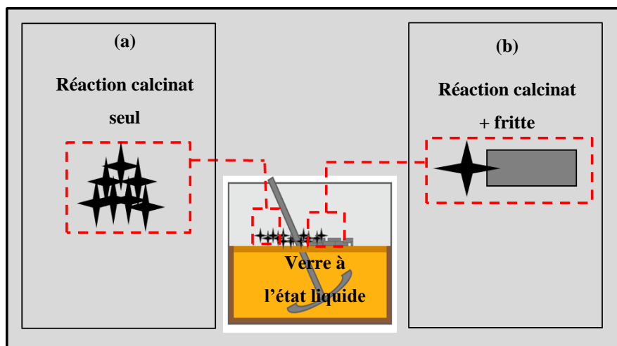
Figure 45 : Schéma récapitulatif des deux modes d'interactions retenus pour l'étude (a) réaction du calcinat maintenu seul en température et (b) réaction entre calcinat et fritte de verre.
