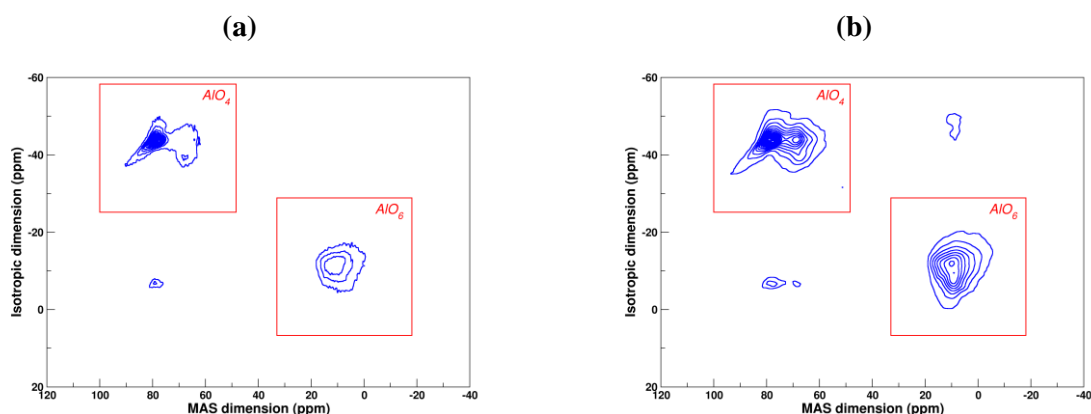
Figure 58 : Mise en évidence de l'hydratation du calcinat C-0Mo-0NdTT par RMN MQMAS ^{27}\text{Al} (a) en août 2014 et (b) en mars 2015.
