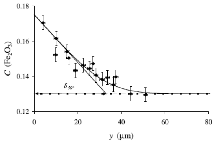
Figure 37 : Profil de concentration de Fe_2O_3 à partir du cristal de spinelle se dissolvant [105].
