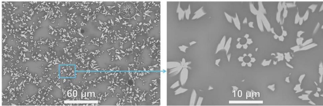
Figure 9 : Cliché MEB mettant en évidence la cristallisation de Ca_2Nd_8(SiO_4)_6O_2 dans un verre simplifié appartenant au système SiO_2-B_2O_3-Na_2O-CaO-Nd_2O_3 après un traitement thermique de 15 minutes à 800 °C [44].
