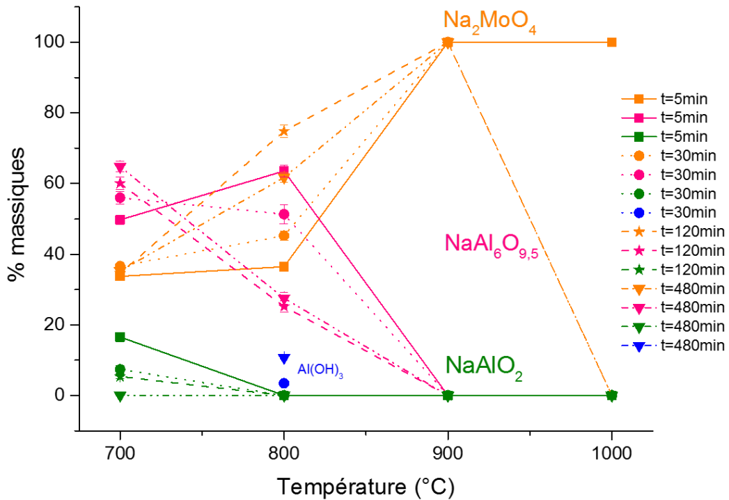
Figure 115 : Evolution des taux de fractions cristallines des phases présentes dans les échantillons de verres à l'issue des tests de réactivité entre la fritte de verre F2 et le calcinat C-20MoTT en fonction du temps et de la température pour un rapport masse fritte/masse verre F/V=0,89 .
