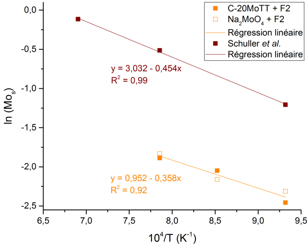
Figure 139 : Mise en évidence du comportement arrhénien de la concentration à saturation en molybdène \text{Mo}_s lors de la dissolution du molybdène dans le verre dans la gamme [800-1000 °C].
