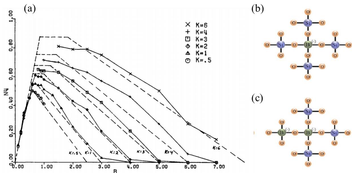
Figure 23 : (a) Variation de N_4 mesurée par RMN en fonction du rapport R=[Na_2O]/[B_2O_3] et K=[SiO_2]/[B_2O_3] . Les traits hachurés correspondent au modèle décrit ci-dessus [34]. (b) Représentation structurale d'une unité reedmergnerite (1 BO_4 pour 4 SiO_4 ) et (c) Représentation structurale d'une unité danburite (1 BO_4 pour 3 SiO_4 et 1 BO_4 ).
